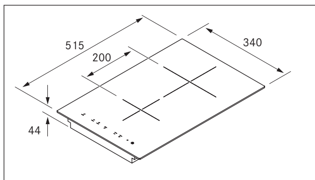
Obr. 3.1 Rozmery prístroja
