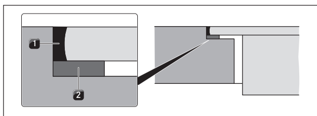
Kuva 5.7 Tiivistenauha uppoasennuksessa
