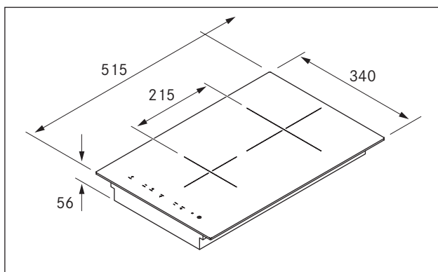
Kuva 3.1 Laitemitat
