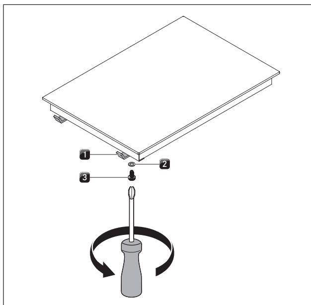
Kuva 5.11 Asennuskannakkeet
