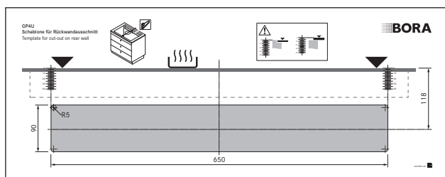
Afb. 5.6 Sjabloon voor achterwanduitsparing
