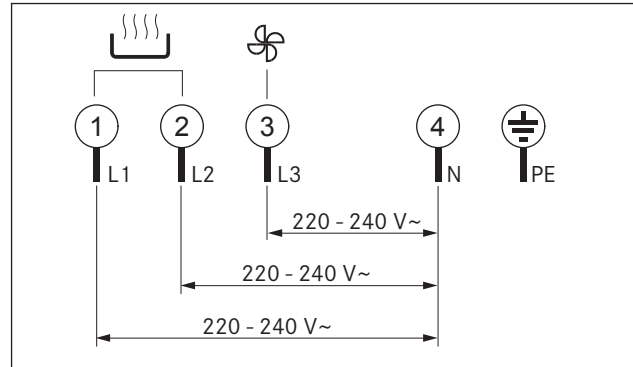
Afb. 5.21 Aansluitschema 3-fasenaansluiting
