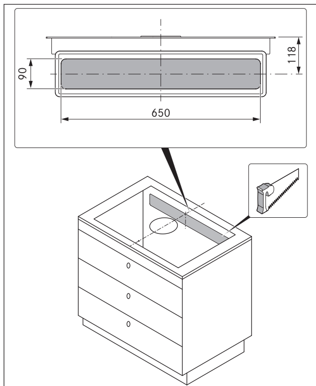
Afb. 5.5 Uitsparing in de achterwand
