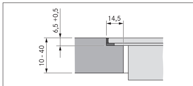
Afb. 5.8 Voegmaat voor vlakinbouw
