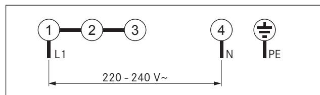
Afb. 5.23 Aansluitschema 1-faseaansluiting
