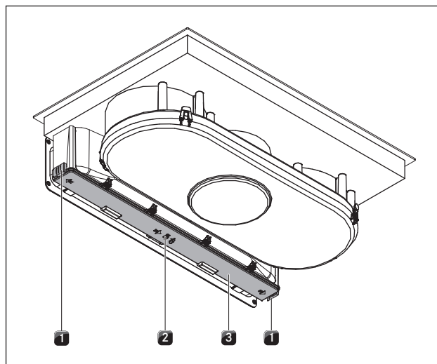
Afb. 12.5 Deksel behuizing actieve-koolfilter ontgrendelen
