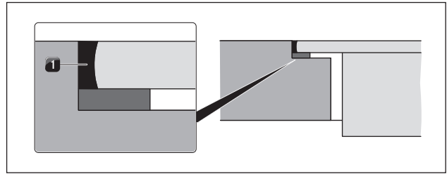
Afb. 5.26 Siliconenkit bij vlakinstallatie
