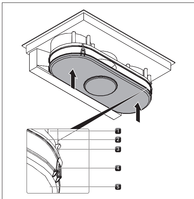
Afb. 12.4 Luchtgeleidingsbehuizing sluiten
