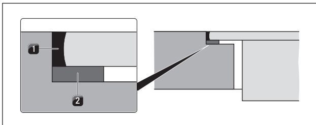
Afb. 5.12 Afdichtingsband bij vlainbouw
