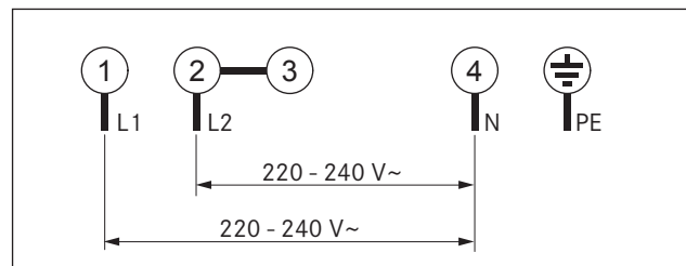
Afb. 5.22 Aansluitschema 2-fasenaansluiting
