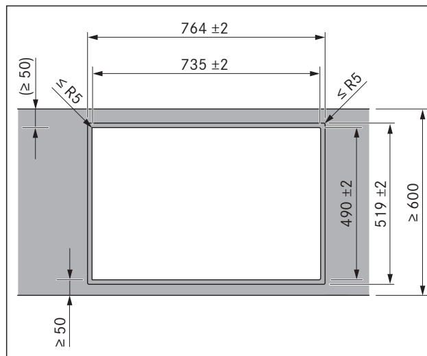
Afb. 5.7 Maten van de uitsparingen voor vlakinbouw
