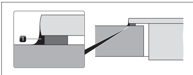
Afb. 5.25 Siliconenkit bij opbouwmontage
