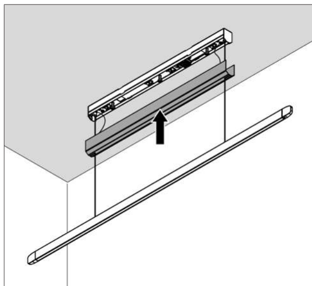
Fig. 5.11 Montaje de la carcasa
