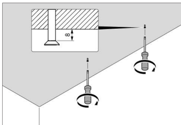
Fig. 5.3 Premontaje del material de fijación
