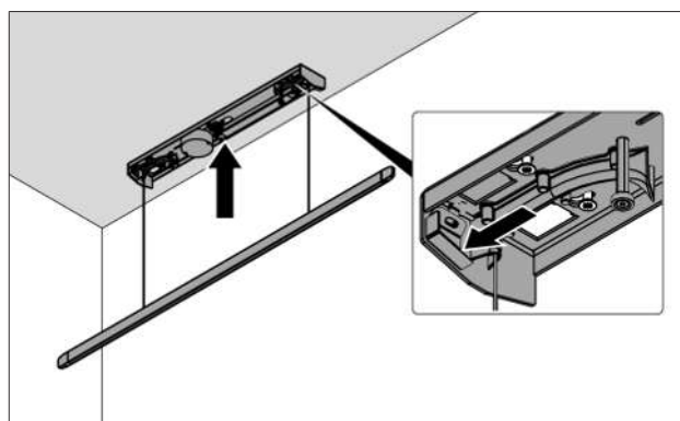
Fig. 5.5 Plasser lampen
