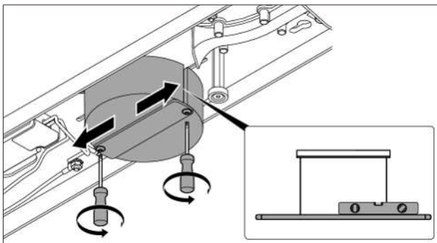
Fig. 5.7 Løsne kabelspolen og juster
