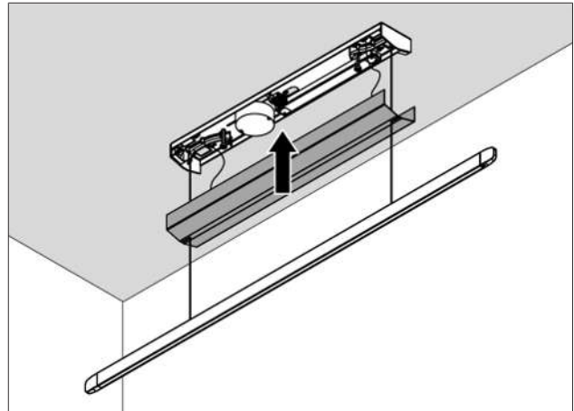
Fig. 5.9 Montere apparatus
