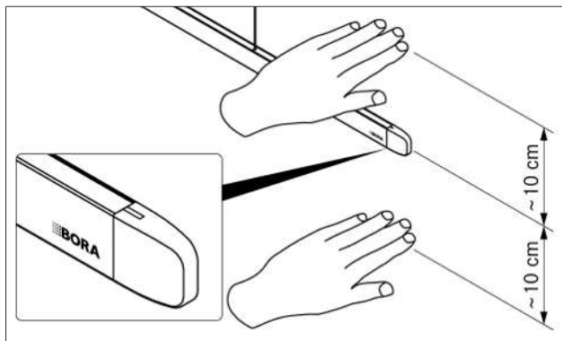
Fig. 6.1 Sensorposisjon
