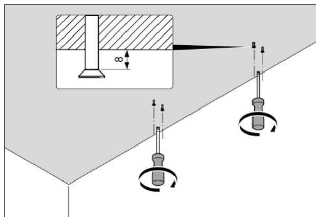
Fig. 5.3 Forhåndsmontér festematerialet
