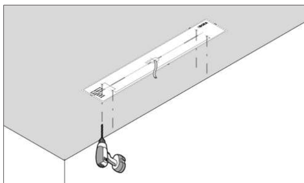
Fig. 5.2 Montering med boremal
