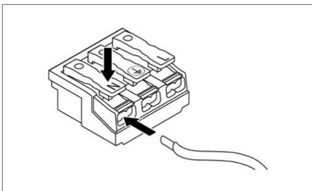
Fig. 5.8 Tilkoblingsklemme
