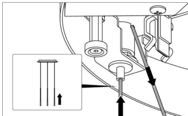
Fig. 5.9 Oppjustere lyskilden
