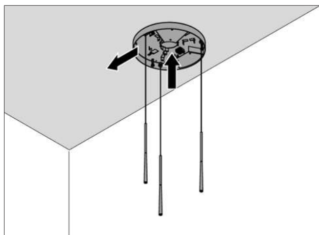
Fig. 5.5 Plasser lampen
