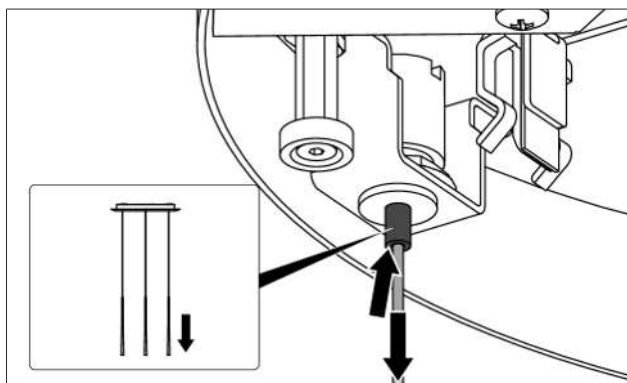
Fig. 5.8 Nedjustere lyskilden
