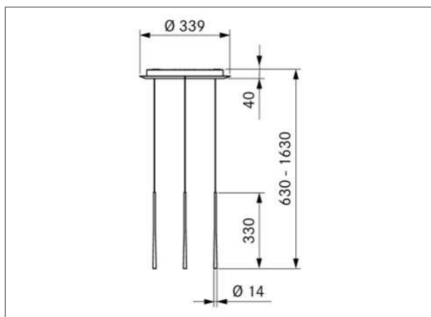
Fig. 3.1 Apparatdimensjoner
