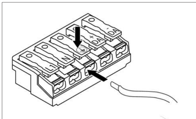
Fig. 5.7 Tilkoblingsklemme
