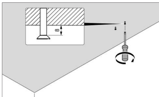
Fig. 5.3 Forhåndsmontér festematerialet
