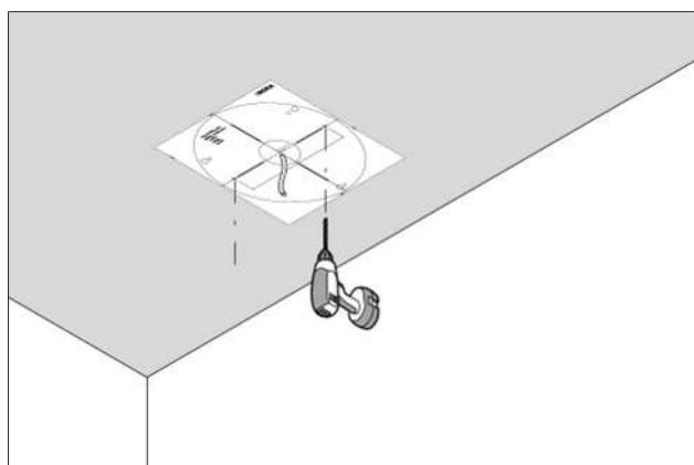
Fig. 5.2 Montering med boremal
