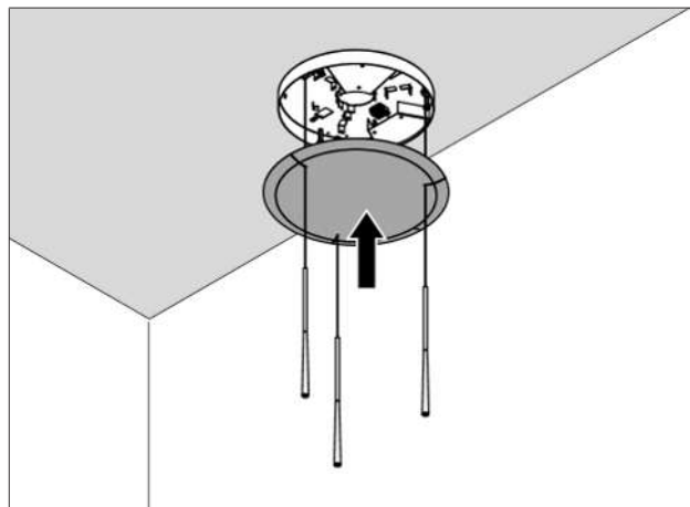
Fig. 5.11 Montere deksel
