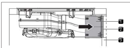
Afb. 9.25 Aansluiting op de achterwand
