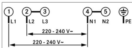
Afb. 9.29 Aansluitschema 2-fasenaansluiting
