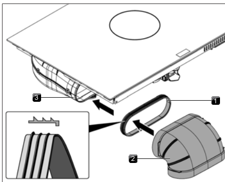
Afb. 9.24 Aansluiting op het kanaalsysteem
