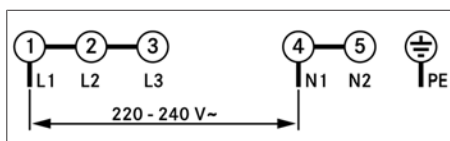
Afb. 9.28 Aansluitschema 1-fasenaansluiting
