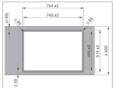
Afb. 9.5 Uitsparingsafmetingen in geval van vlakinbouw
