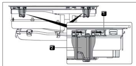
Afb. 9.19 Montageklemmen aanbrengen
