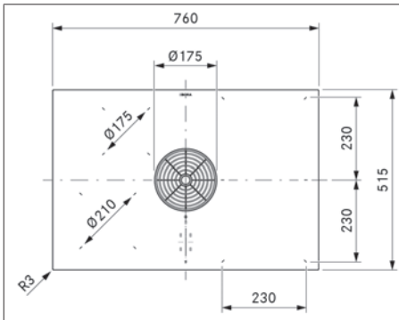
Afb. 3.4 PURMU toestelafmetingen bovenaanzicht
