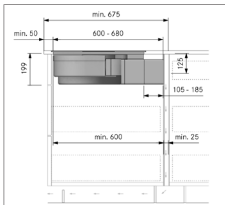
Afb. 9.14 Inbouwmaten bij recirculatie - montagevariant A, werkbladdiepte vanaf 675 mm
