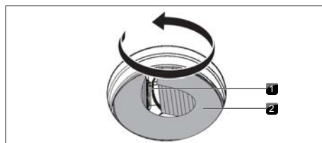
Afb. 7.4 Actieve-koolfilter uit de filterbehuizing draaien
