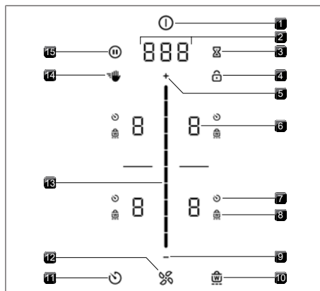
Afb. 4.4 Bedieningspaneel
