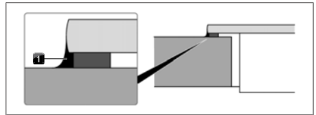
Afb. 9.35 Siliconenkit bij opbouwmontage
