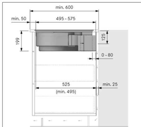
Afb. 9.13 Inbouwmaten bij recirculatie, montagevariant A
