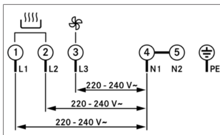
Afb. 9.27 Aansluitschema 3-fasenaansluiting
