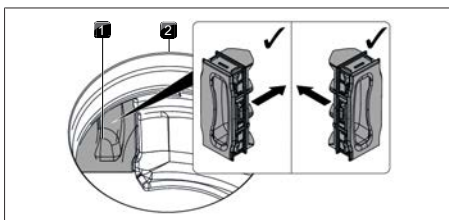
Afb. 7.9 Filtervervangingsklep plaatsen
