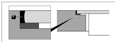
obr. 11.36 Silikonová těsnicí hmota při plošně zarovnané montáži
