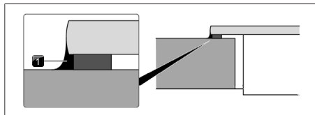
obr. 11.35 Silikonová těsnicí hmota při montáži na povrch
