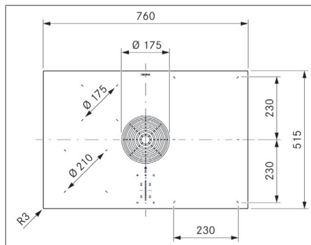
obr. 3.4 Rozměry produktu PURMU2/R – pohled shora
