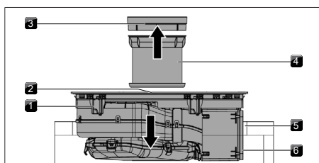
obr. 11.20 Upevnění varné desky do středu
