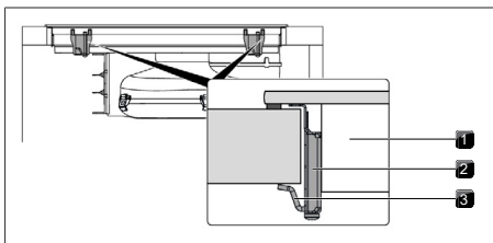
obr. 11.23 Upevnění varné desky do středu
