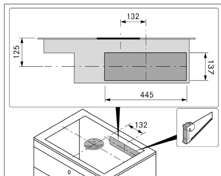
obr. 11.11 Výřez v zadní stěně
