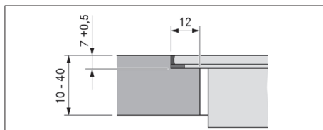
obr. 11.6 Rozměr drážky pro plošně zarovnanou montáž
