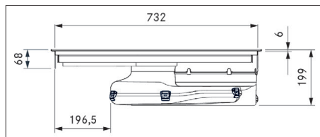
obr. 3.5 Rozměry produktu PURMU2/R – pohled zepředu
