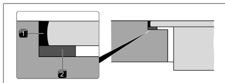
obr. 11.18 Těsnicí páska při plošně zarovnané montáži
