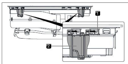
obr. 11.19 Umístění montážních svorek
