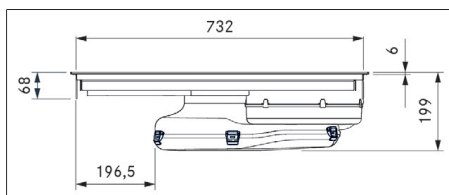
obr. 3.2 Rozměry produktu PURMA2/R – pohled zepředu
