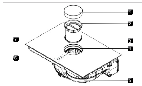
obr. 4.1 Uspořádání
