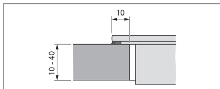
obr. 11.8 Rozměry podkladu pro montáž na povrch
