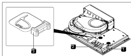
obr. 11.30 Elektrické přípojky varné desky
