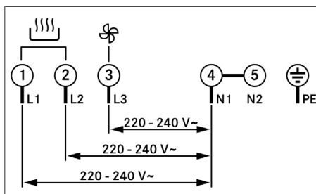
obr. 11.27 Schéma zapojení 3fázové přípojky
