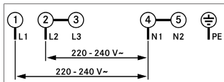
obr. 11.29 Schéma zapojení 2fázové přípojky
