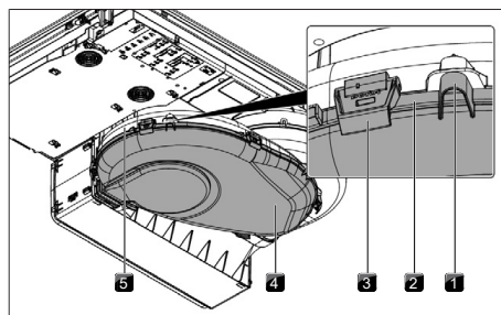
obr. 9.3 Skříň ventilace
