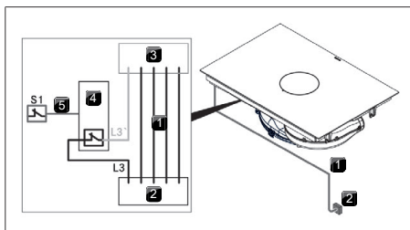
obr. 11.26 Schéma zapojení s externím spínacím kontaktem
