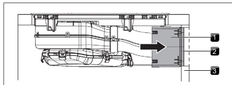
obr. 11.25 Přípojka k zadní stěně
