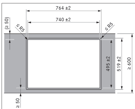
obr. 11.5 Rozměry výřezu pro plošně zarovnanou montáž
