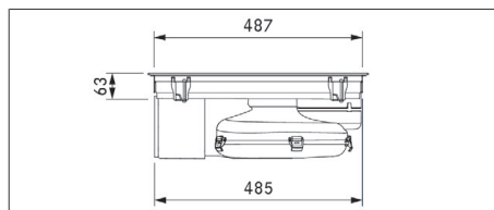
obr. 3.6 Rozměry produktu PURMU2/R – pohled z boku
