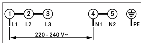
obr. 11.28 Schéma zapojení 1fázové přípojky
