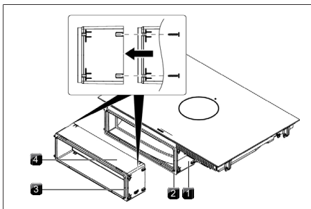
obr. 11.15 Nadstavení teleskopického výsuvu
