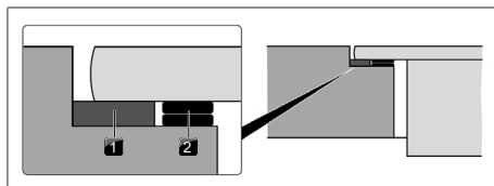
Fig. 11.22 Højdeudligningsplader
