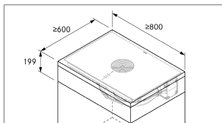
Fig. 11.4 Møbel mindstemål
