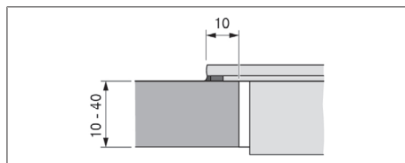
Fig. 11.8 Påsætningsmål til overflademontering
