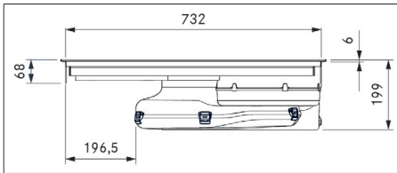
Fig. 3.5 PURMU2/R - enhedens mål set forfra
