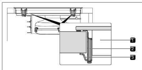
Fig. 11.23 Fastgøring af kogepladen i midten
