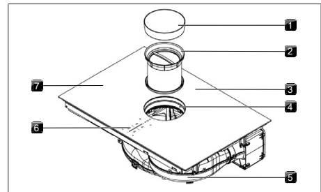
Fig. 4.1 Opbygning
