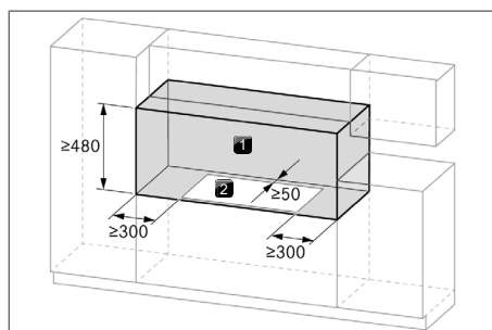
Fig. 11.3 Krævet frirum
