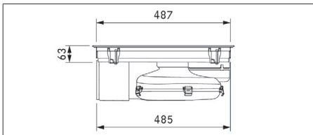
Fig. 3.6 PURMU2/R - enhedens mål set fra siden
