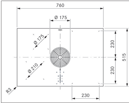
Fig. 3.4 PURMU2/R - enhedens mål set fra oven
