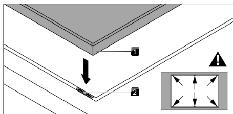
Fig. 11.21 Placering af højdeudligningspladerne
