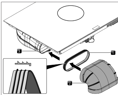
Fig. 11.24 Tilslutning til kanalsystem
