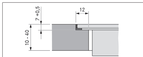
Fig. 11.6 Falsmål til planimet monteret
