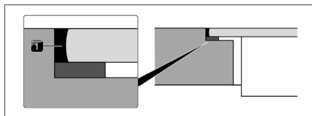
Fig. 11.36 Silikonetætningsmasse ved planlimet montering
