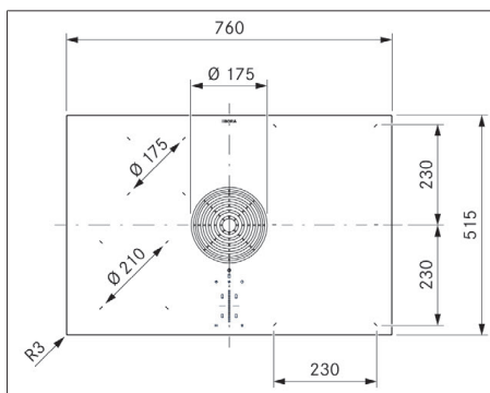
Fig. 3.1 PURMA2/R - enhedens mål set fra oven
