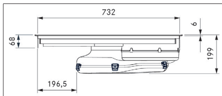
Fig. 3.2 PURMA2/R - enhedens mål set forfra
