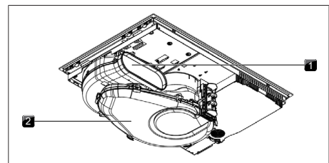
Fig. 4.2 Udsugningsvariant set bagfra
