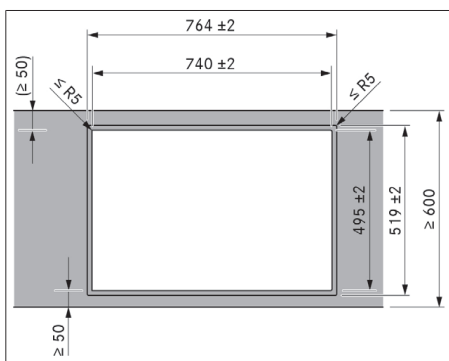
Fig. 11.5 Udskæringsmål til planlimet montering
