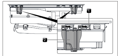
Abb. 11.19 Montageklemmen anbringen
