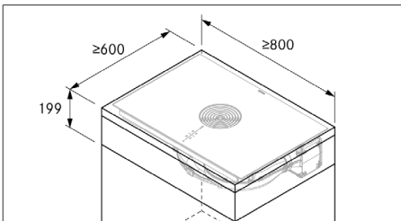
Abb. 11.4 Möbel-Mindestmaße
