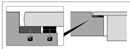
Abb. 11.22 Höhenausgleichsplatten
