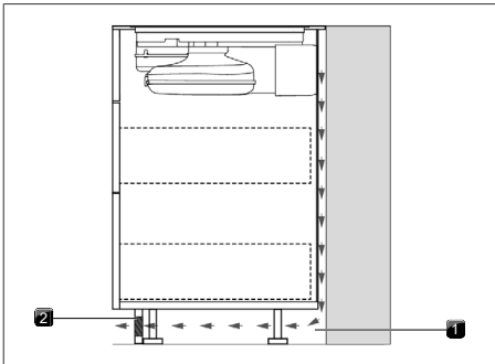
Abb. 11.10 Rückströmöffnung im Sockelbereich
