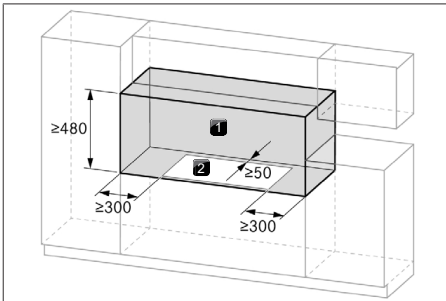
Abb. 11.3 Erforderlicher Freiraum
