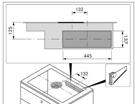
Abb. 11.11 Rückwand-Ausschnitt
