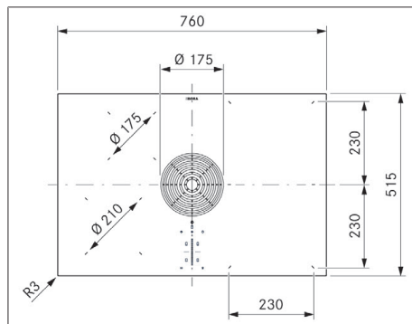
Abb. 3.4 PURMU2/R Gerätemaße Draufsicht
