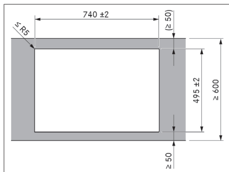
Abb. 11.7 Ausschnittsmaße für Aufsatzmontage
