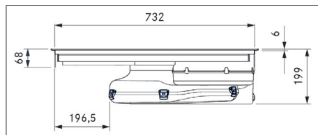
Abb. 3.5 PURMU2/R Gerätemaße Vorderansicht
