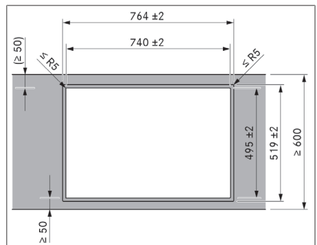
Abb. 11.5 Ausschnittsmaße für flächenbündige Montage
