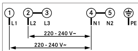
Abb. 11.29 Anschlusschema 2-Phasen-Anschluss
