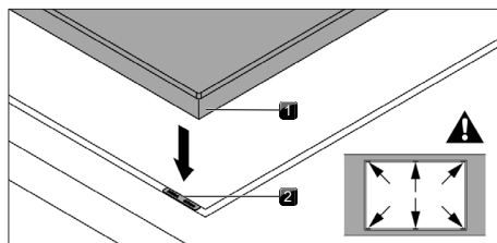
Abb. 11.21 Positionierung der Höhenausgleichsplatten
