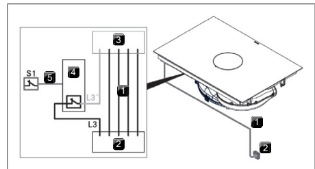
Abb. 11.26 Anschlussschema mit externem Schaltkontakt
