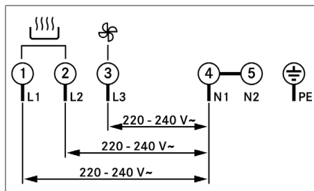
Abb. 11.27 Anschlusschema 3-Phasen-Anschluss
