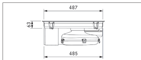
Abb. 3.6 PURMU2/R Gerätemaße Seitenansicht
