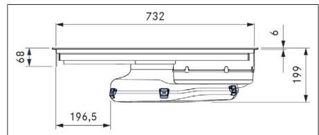
Abb. 3.2 PURMA2/R Gerätemaße Vorderansicht
