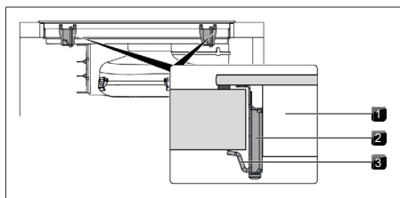
Abb. 11.23 Kochfeld mittig befestigen
