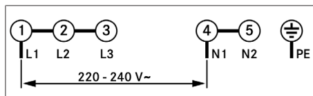
Abb. 11.28 Anschlusschema 1-Phasen-Anschluss
