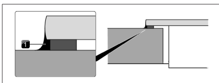
Kuva 11.35 Silikoniitiivistysmassa pinta-asennuksessa
