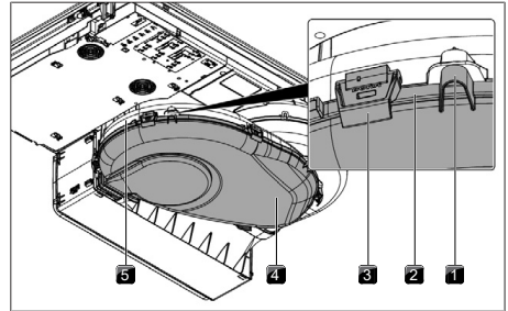
Kuva 9.3 Ilmanohjaukotelon
