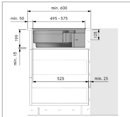
Kuva 11.16 Asennusmitat kiertoilma-asennuksessa B, työtason syvyys 600 mm
