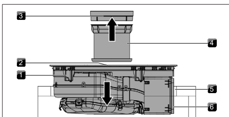
Kuva 11.20 Keittotason asettaminen keskelle
