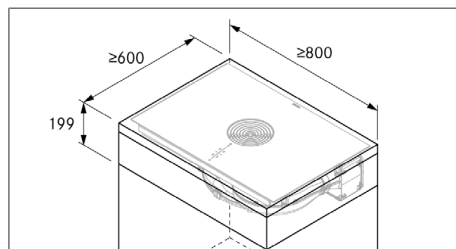
Kuva 11.4 Kalusteen vähimmäismitat
