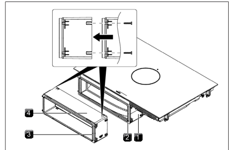
Kuva 11.15 Ulosvedettävän osan pidennys
