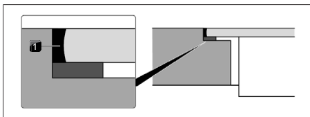
Kuva 11.36 Silikoniitiivistysmassa uppoasennuksessa
