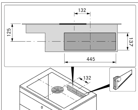
Kuva 11.11 Takaseinän aukko
