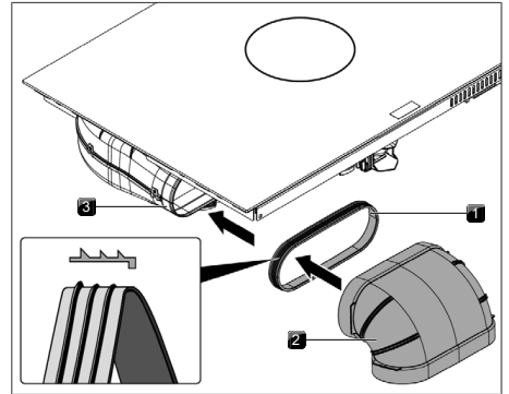
Kuva 11.24 Liittäminen kanavajärjestelmään
