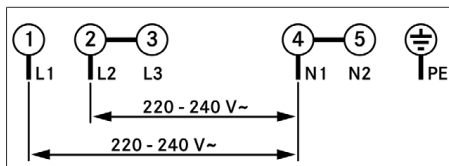
Kuva 11.29 Liitäntäkaavio - 2-vaiheiliitäntä
