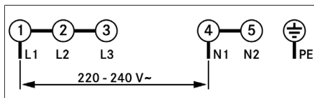
Kuva 11.28 Liitäntäkaavio - 1-vaiheiliitäntä
