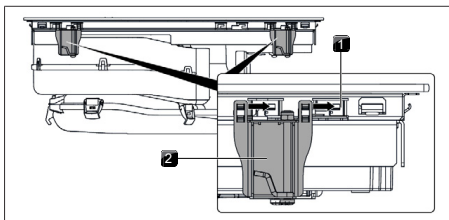
Kuva 11.19 Kiinnittimien kiinnittäminen
