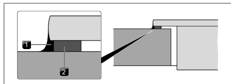
Kuva 11.17 Tiivistenauha pinta-asennuksessa
