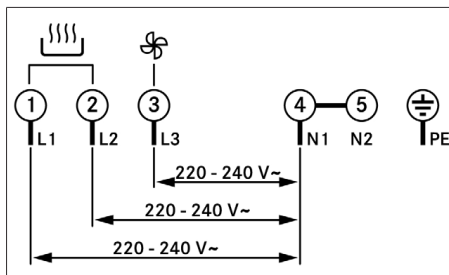
Kuva 11.27 Liitäntäkaavio - 3-vaiheiliitäntä
