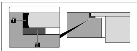
Kuva 11.18 Tiivistenauha uppoasennuksessa
