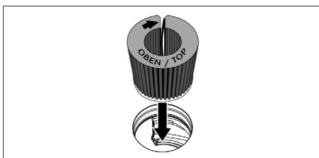
Kuva 9.8 Hajusuodattimen asettaminen tuloaukkoon
