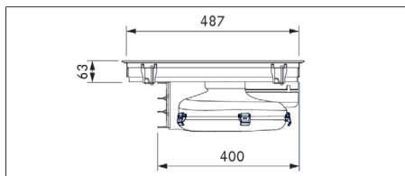
Kuva 3.3 Laitemitat PURMA2/R sivukuva
