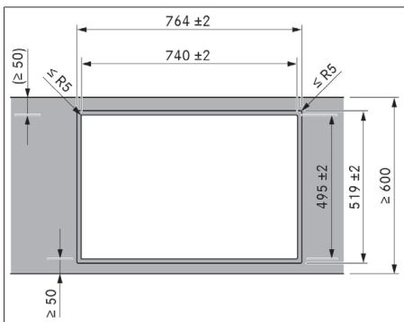
Kuva 11.5 Asennusaukon mitat uppoasennusta varten
