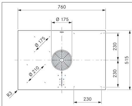
Kuva 3.1 Laitemitat PURMA2/R kuva ylhäältä
