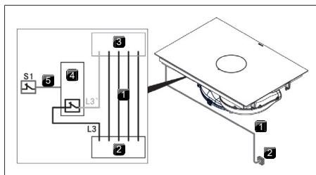
Kuva 11.26 Liitäntäkaavio, ulkoinen kytkin
