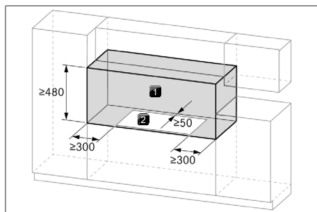
Kuva 11.3 Tarvittava vapaa tila
