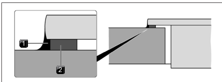
Afb. 11.17 Afdichtingsband bij opbouwmontage
