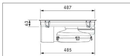
Afb. 3.6 PURMU2/R toestelafmetingen zijaanzicht
