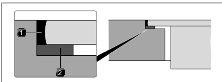
Afb. 11.18 Afdichtingsband bij vlainbouw
