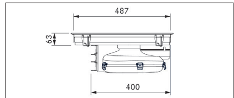
Afb. 3.3 PURMA2/R toestelafmetingen zijaanzicht
