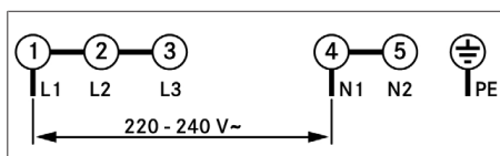
Afb. 11.28 Aansluitschema 1-faseaansluiting
