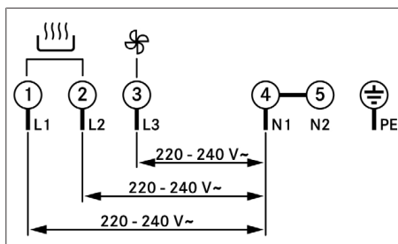
Afb. 11.27 Aansluitschema 3-faseaansluiting
