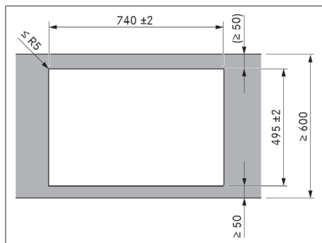
Afb. 11.7 Uitsparingsafmetingen in geval van opbouwmontage
