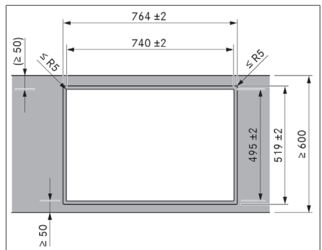
Afb. 11.5 Uitsparingsafmetingen in geval van vlakinbouw
