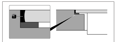
Afb. 11.36 Siliconenkit bij vlakinbouw
