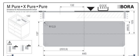
Afb. 11.12 Sjabloon voor achterwanduitsparing
