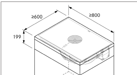
Afb. 11.4 Minimale meubelafmetingen
