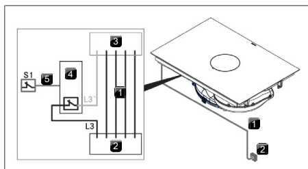
Afb. 11.26 Aansluitschema met extern schakelcontact
