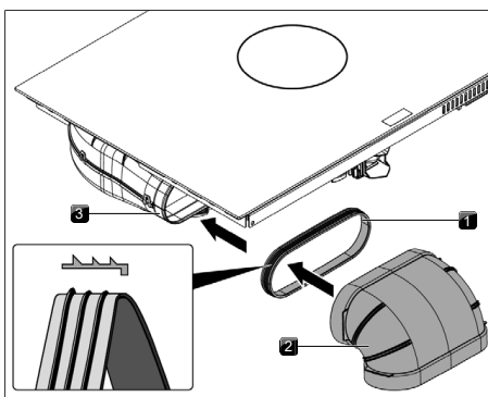
Afb. 11.24 Aansluiting op het kanaalsysteem
