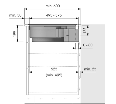
Afb. 11.13 Inbouwmaten bij recirculatie, montagevariant A
