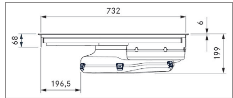
Afb. 3.2 PURMA2/R toestelafmetingen vooraanzicht
