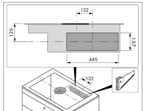
Afb. 11.11 Achterwanduitsparing
