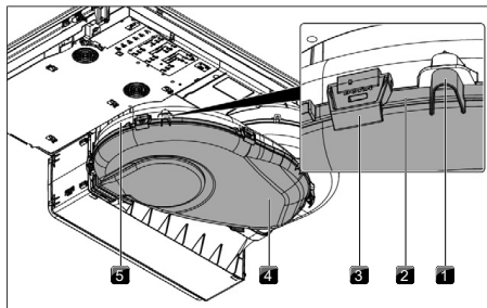
Afb. 9.3 Luchtgeleidingsbehuizing
