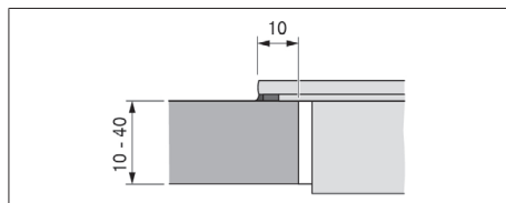
Afb. 11.8 Oplegmaat voor opbouwmontage
