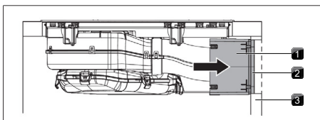
Afb. 11.25 Aansluiting op de achterwand
