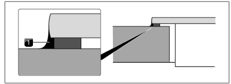
Afb. 11.35 Siliconenkit bij opbouwmontage
