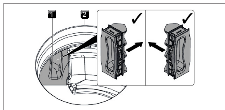
Afb. 9.10 Filtervervangingsklep plaatsen
