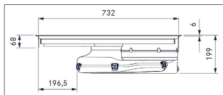
Afb. 3.5 PURMU2/R toestelafmetingen vooraanzicht
