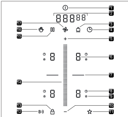
Afb. 4.4 Bedieningspaneel
