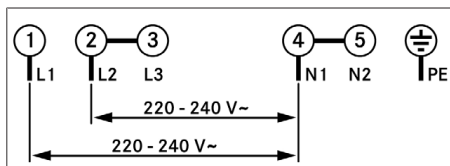
Afb. 11.29 Aansluitschema 2-faseaansluiting
