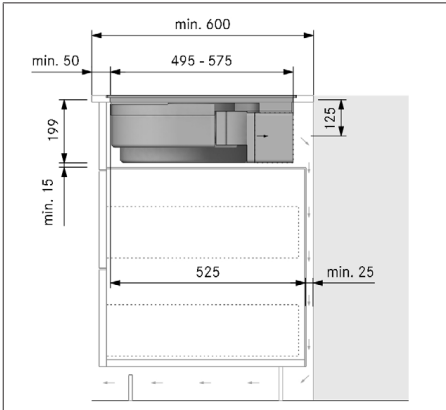
Afb. 11.16 Inbouwmaten bij recirculatie - montagevariant B, werkbladdiepte 600 mm
