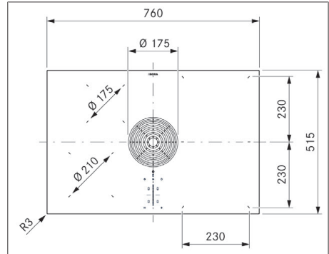
Afb. 3.1 PURMA2/R toestelafmetingen bovenaanzicht
