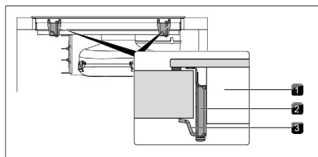
Afb. 11.23 Centrale bevestiging kookveld
