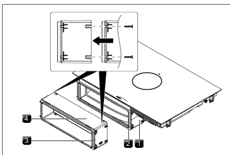
Afb. 11.15 Verlenging telescopisch kanaal
