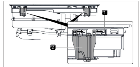
Afb. 11.19 Montageklemmen aanbrengen
