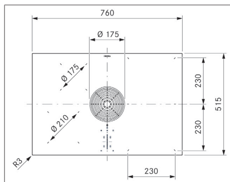
Afb. 3.4 PURMU2/R toestelafmetingen bovenaanzicht
