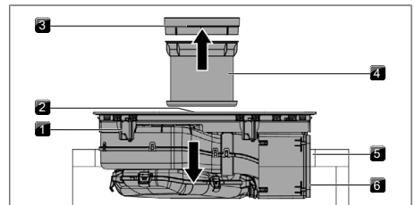
Afb. 11.20 Centrale plaatsing kookveld
