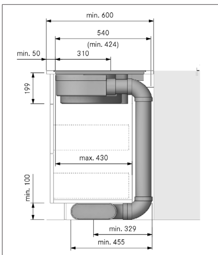
Afb. 11.9 Inbouwmaten luchtafvoer, werkbladdiepte 600 mm
