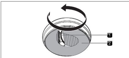
Afb. 9.5 Geurfilter uit de filterbehuizing draaien
