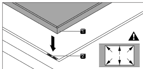
Afb. 11.21 Positionering van de vulplaatjes
