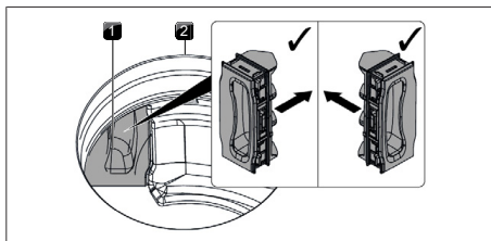
Rys. 9.10 Wkładanie kłapy wymiany filtra
