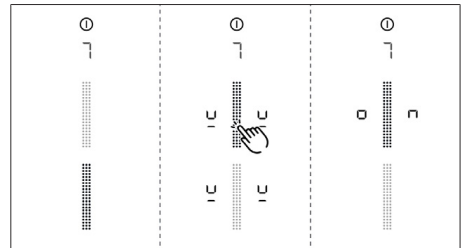
Rys. 8.8 Punkt menu 7: Stałe rozpoznawanie naczynia
