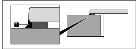
Rys. 11.35 Masa silikonowa przy montażu elementu z uskokiem
