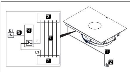
Rys. 11.26 Schemat podłączenia z zewnętrznym stykiem przełączającym
