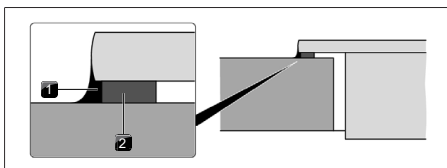
Rys. 11.17 Taśma uszczelniająca przy montażu elementu z uskokiem
