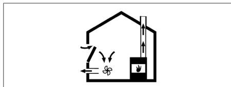
Rys. 11.2 Montaż instalacji z odprowadzeniem powietrza na zewnątrz – prawidłowy
