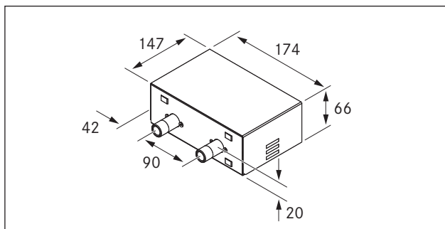
Afb. 3.2 Afmetingen schakelkast
