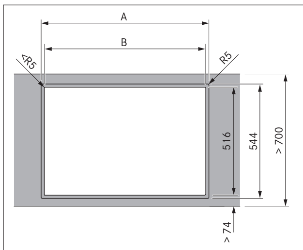
Afb. 5.3 Vlakbouw
