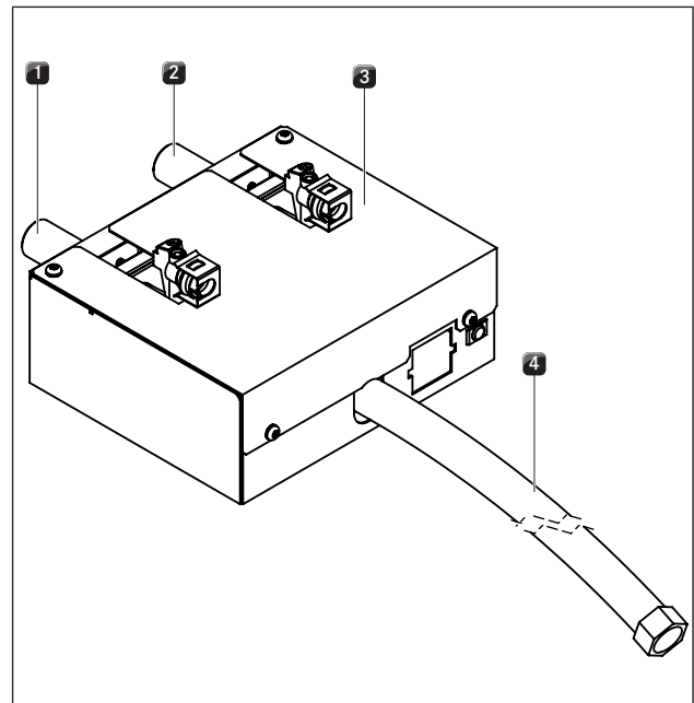
Afb. 4.1 Schakelkast
