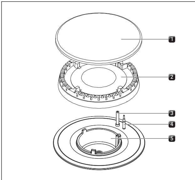
Afb. 8.1 Opbouw gasbrander
