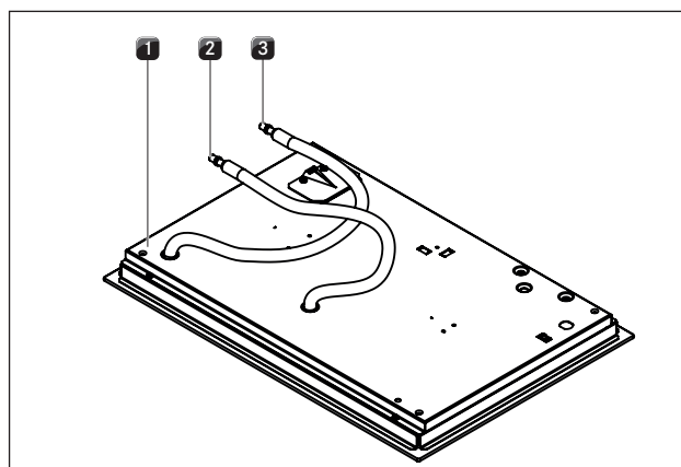
Afb. 5.1 Kookveld
