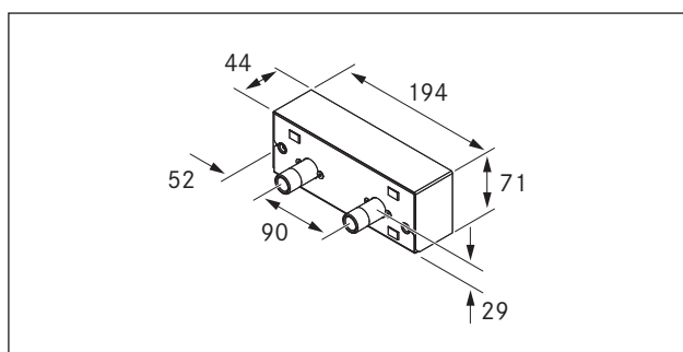
Fig. 3.2 Styreboksmål
