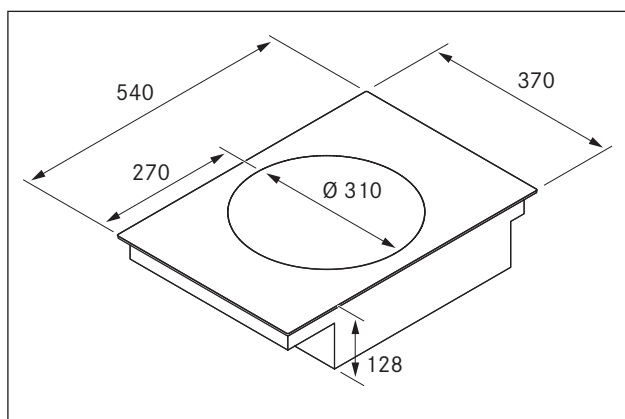
Fig. 3.1 Dimensioni apparecchio
