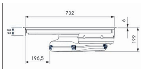
obr. 3.2 Rozměry spotřebiče PURA – pohled zepředu
