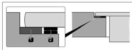
obr. 9.22 Podložky k nastavení výšky
