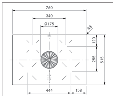
obr. 3.4 Rozměry spotřebiče PURU – pohled shora
