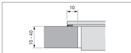
obr. 9.8 Rozměry podkladu pro montáž na povrch
