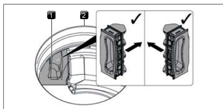
obr. 7.9 Nasazení výměnné klapky filtru
