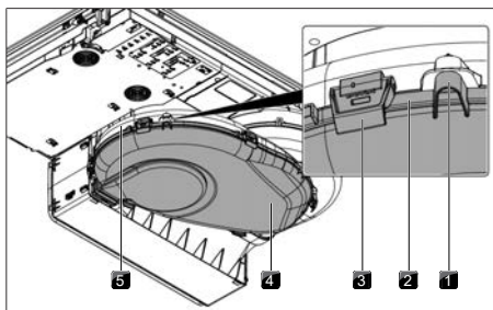
obr. 7.2 Skříň ventilace
