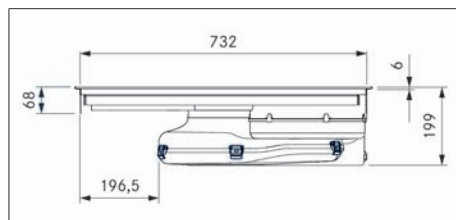
obr. 3.5 Rozměry spotřebiče PURU – pohled zepředu
