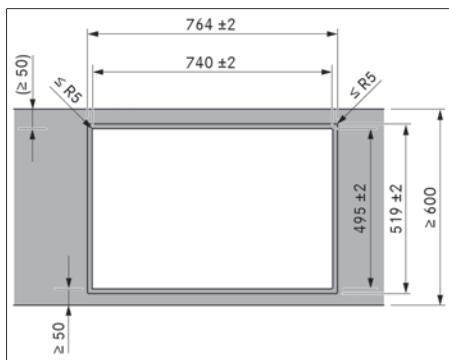
obr. 9.5 Rozměry výřezu pro plošně zarovnanou montáž
