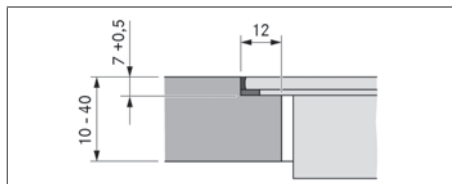
obr. 9.6 Rozměr drážky pro plošně zarovnanou montáž
