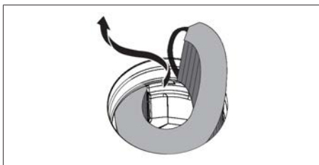
obr. 7.5 Vyjmutí filtru s aktivním uhlím z otvoru přívodní trysky
