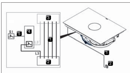
obr. 9.26 Schéma zapojení s externím spínacím kontaktem
