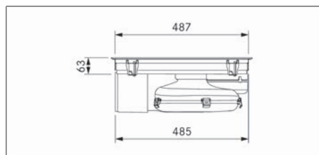
obr. 3.6 Rozměry spotřebiče PURU – pohled z boku
