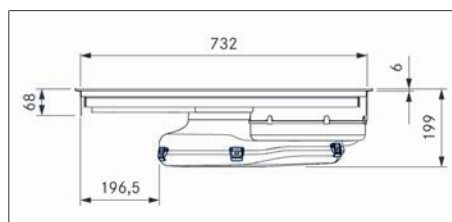
Fig. 3.2 PURA dimensioni apparecchio vista frontale
