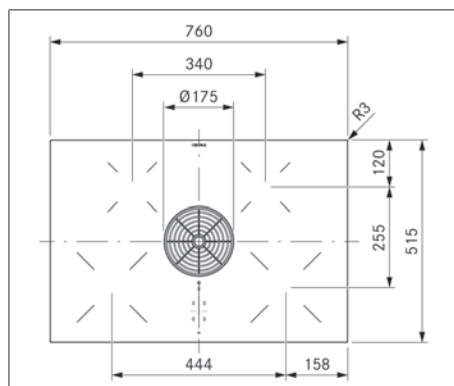
Fig. 3.4 PURU dimensioni apparecchio visto da sopra
