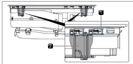
Fig. 9.19 Applicare i morsetti di montaggio
