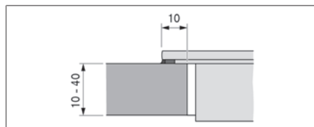
Fig. 9.8 Misura d'appoggio per montaggio in battuta
