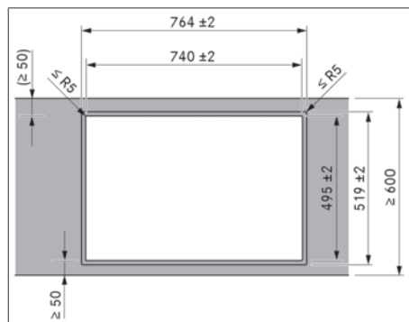
Fig. 9.5 Dimensioni intaglio per montaggio a filo
