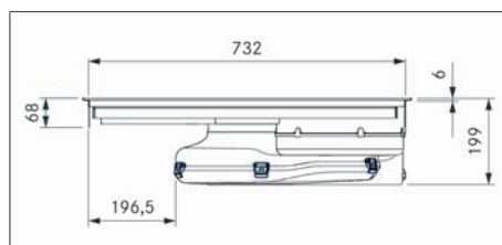
Fig. 3.5 PURU dimensioni apparecchio vista frontale
