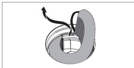
Fig. 7.5 Rimuovere il filtro al carbone attivo dall'apertura immissione aria
