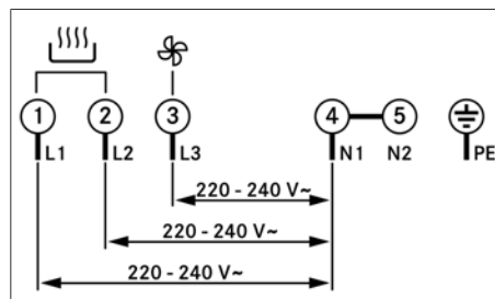
Fig. 9.27 Schema di collegamento, collegamento trifase
