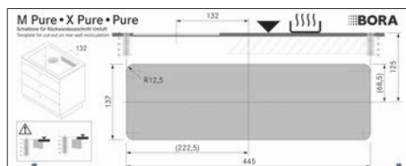
Fig. 9.12 Maschera per intaglio parete posteriore
