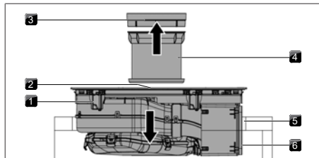
Fig. 9.20 Inserire il piano cottura nel centro
