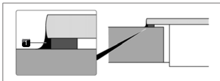
Fig. 9.35 Pasta sigillante al silicone per montaggio in battuta
