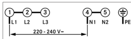
Fig. 9.28 Schema di collegamento, collegamento monofase
