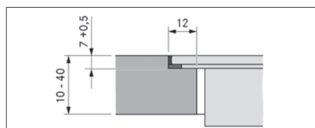
Fig. 9.6 Dimensioni dell'incassatura per montaggio a filo piano
