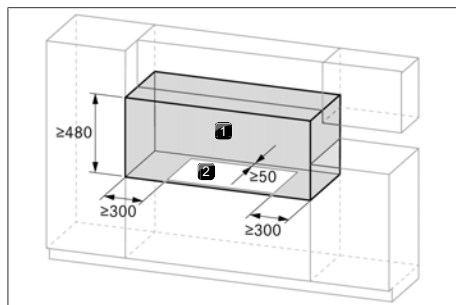
Fig. 9.3 Spazio libero necessario
