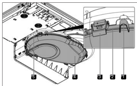
Fig. 7.2 Alloggiamento conduttura aria
