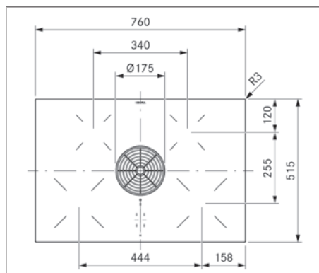
Fig. 3.1 PURA dimensioni apparecchio vista dall'alto
