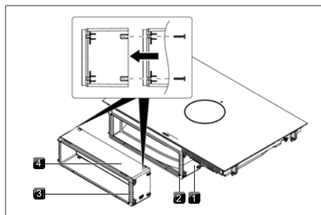
Fig. 9.15 Estensione della prolunga telescopica
