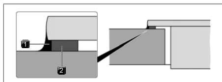
Fig. 9.17 Nastro a tenuta per montaggio in battuta
