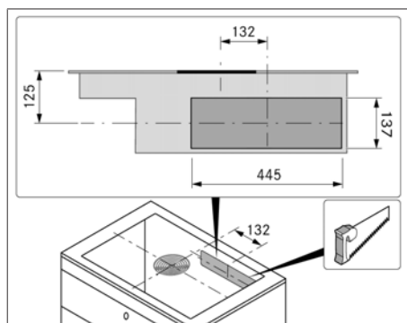
Fig. 9.11 Sezione parete posteriore
