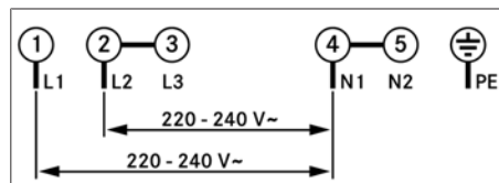
Fig. 9.29 Schema di collegamento, collegamento bifase
