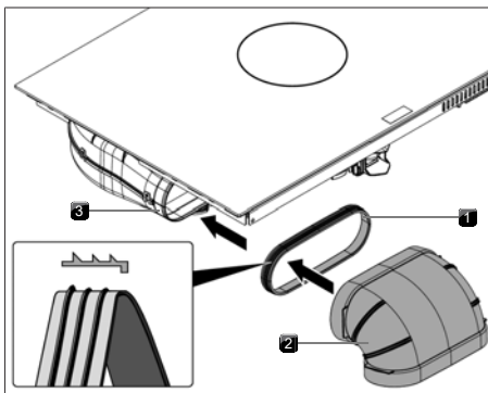
Fig. 9.24 Connessione al sistema di canali
