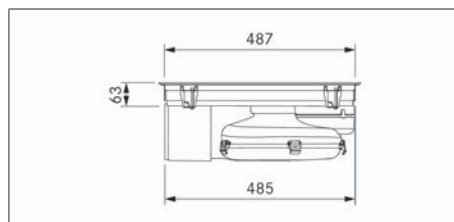
Fig. 3.6 PURU dimensioni apparecchio visto laterale
