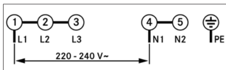
Rys. 9.28 Schemat podłączenia, przyłącze 1-fazowe
