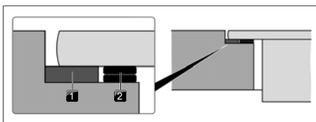
Rys. 9.22 Podkładki wyrównujące
