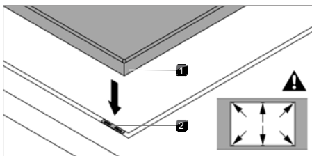
Rys. 9.21 Umieszczenie podkładek wyrównujących
