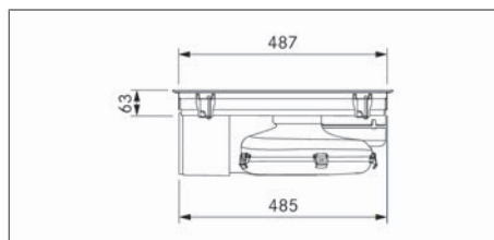
Rys. 3.6 PURU Wymiary urządzenia - widok z boku
