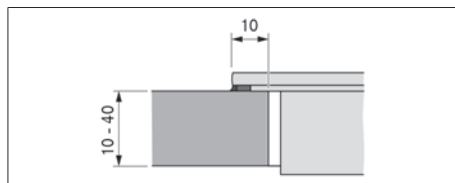
Rys. 9.8 Wymiary podparcia dla montażu elementu z uskokiem
