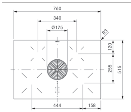
Rys. 3.1 PURA Wymiary urządzenia – widok z góry
