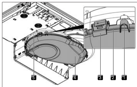
Rys. 7.2 Obudowa kanału powietrza
