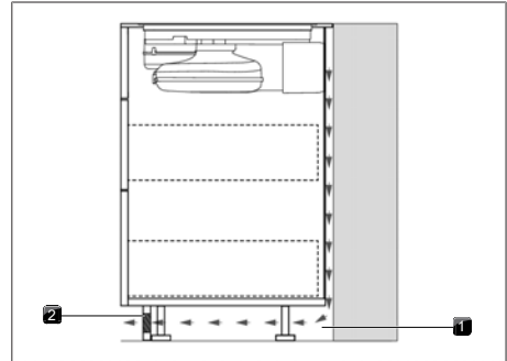
Rys. 9.10 Otwór na strumień zwrotny w obszarze cokołu
