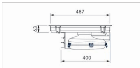
Rys. 3.3 PURA Wymiary urządzenia – widok z boku
