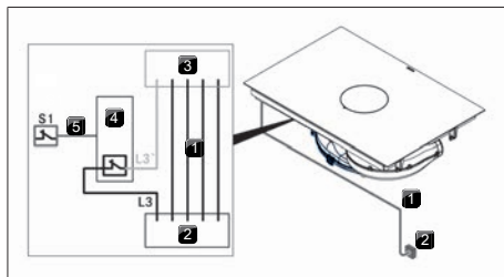
Rys. 9.26 Schemat podłączenia z zewnętrznym stykiem przełączającym
