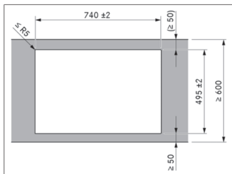
Rys. 9.7 Wymiary wycięcia dla montażu elementu z uskokiem
