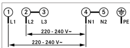
Rys. 9.29 Schemat podłączenia, przyłącze 2-fazowe
