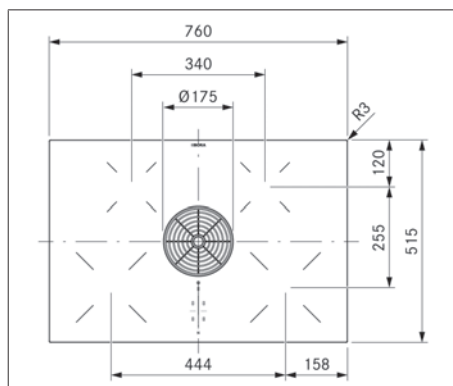
Rys. 3.4 PURU Wymiary urządzenia - widok z góry
