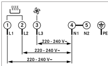
Rys. 9.27 Schemat podłączenia, przyłącze 3-fazowe
