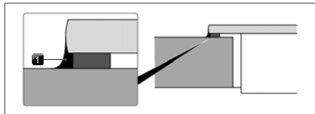
Rys. 9.35 Masa silikonowa przy montażu elementu z uskokiem
