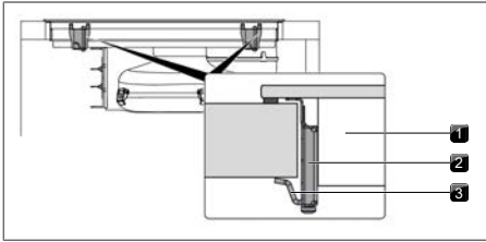
Rys. 9.23 Centralne mocowanie płyty grzewczej
