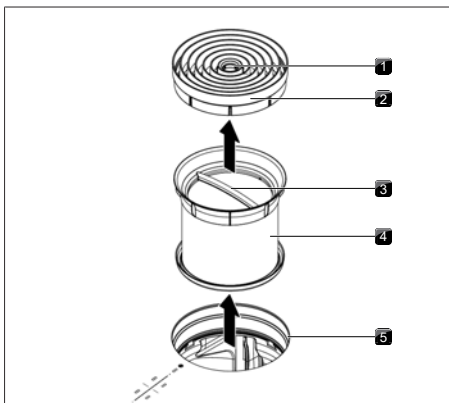
Rys. 7.1 Demontaż komponentów
