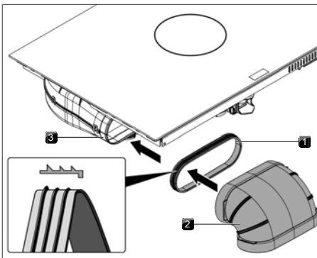
Rys. 9.24 Podłączenie do systemu kanałów
