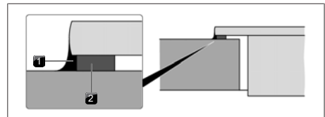
Rys. 9.17 Taśma uszczelniająca przy montażu elementu z uskokiem
