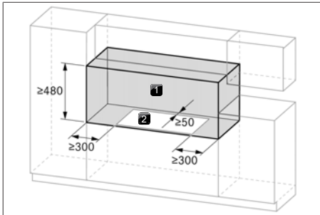
Rys. 9.3 Wymagane odstępy
