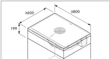
Rys. 9.4 Minimalne wymiary mebli
