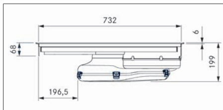
Rys. 3.2 PURA Wymiary urządzenia – widok z przodu
