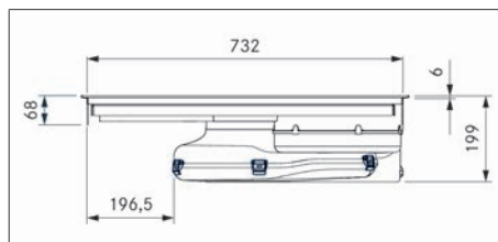
Rys. 3.5 PURU Wymiary urządzenia - widok z przodu
