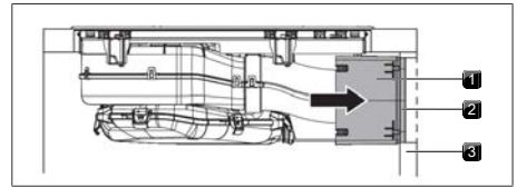
Rys. 9.25 Połączenie z tylną ścianą
