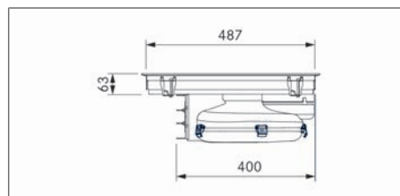
Sl. 3.3 Dimenzije naprave PURA, pogled s strani
