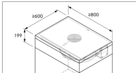
Sl. 9.4 Najmanjše dimenzije pohoštva
