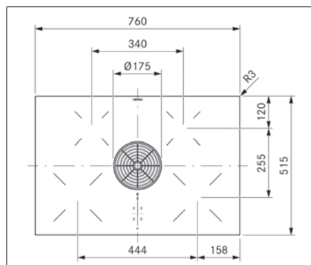
Sl. 3.1 Dimenzije naprave PURA, pogled od zgoraj
