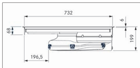
Sl. 3.5 Dimenzije naprave PURU, pogled od spredaj
