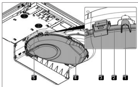
Sl. 7.2 Ohišje zračnega kanala
