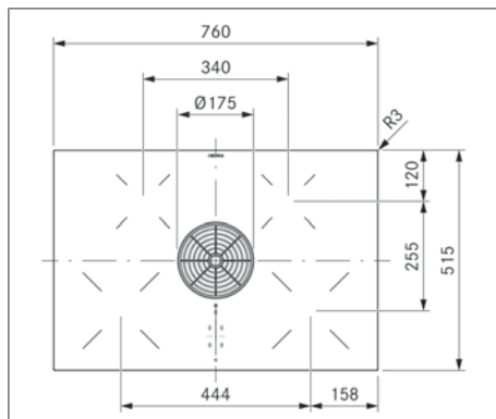
Sl. 3.4 Dimenzije naprave PURU, pogled od zgoraj
