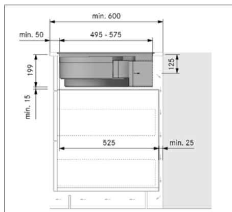
Sl. 9.16 Dimenzije vgradnje pri različici montaže B z obtočnim zakrnom, globina delovne plošče 600 mm
