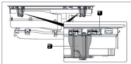
Sl. 9.19 Namestitev montažnih sponk
