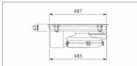
Sl. 3.6 Dimenzije naprave PURU, pogled s strani
