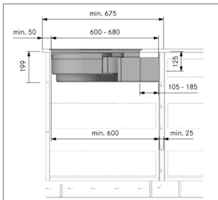
Sl. 9.14 Dimenzije vgradnje pri različici montaže A z obtočnim zrakom, globina delovne plošče od 675 mm
