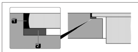
Sl. 9.18 Trak za tesnjenje pri montaži v isti ravni s površino
