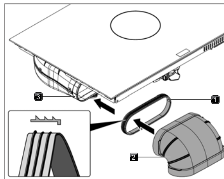
Sl. 9.24 Priključitev na sistem kanala
