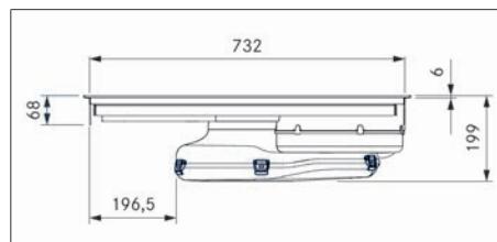
Sl. 3.2 Dimenzije naprave PURA, pogled od spredaj
