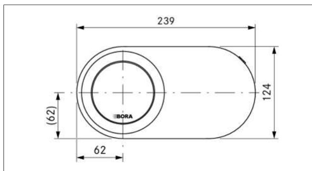
Afb. 3.2 Bovenaanzicht QVac
