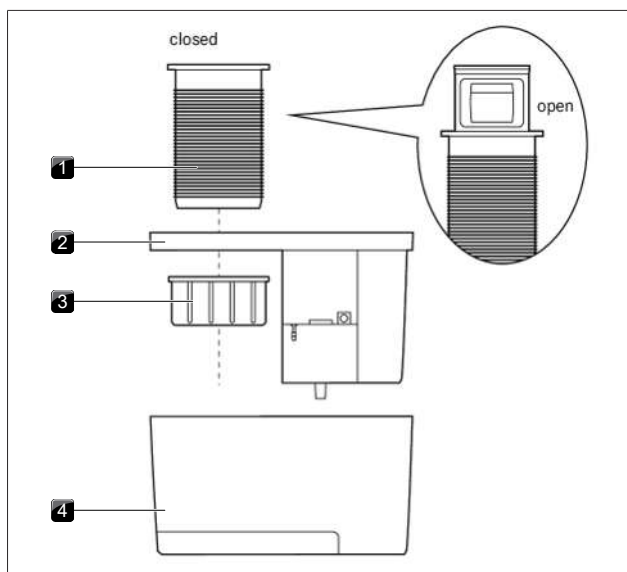
Afb. 8.1 Onderdelen
