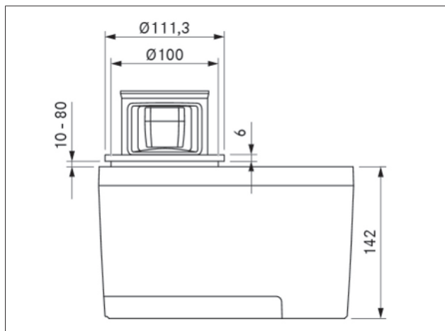
Afb. 3.1 Vooraanzicht QVac
