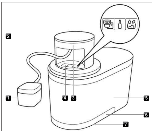
Afb. 4.1 Opbouw
