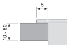
Afb. 8.5 Oplegmaat voor opbouwmontage
