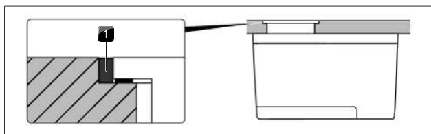
Afb. 8.21 Pop-up unit afwerken
