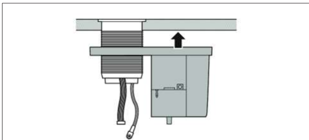
Afb. 8.15 Basisstation plaatsen
