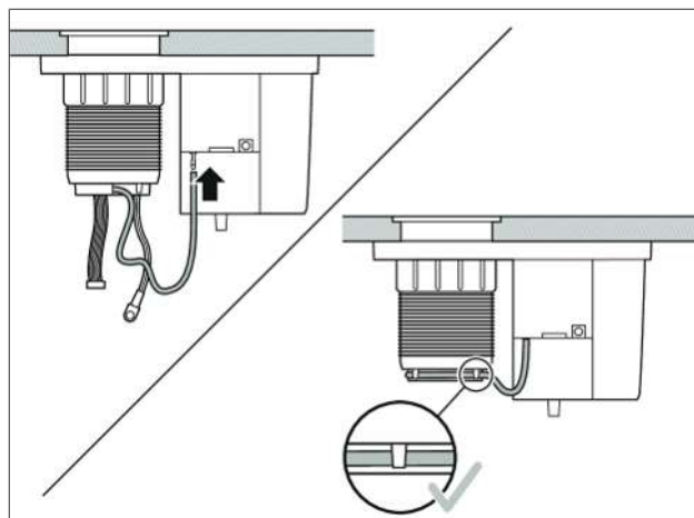
Afb. 8.17 De vacuümslang aansluiten en vastzetten
