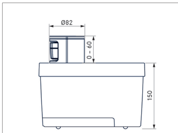
Afb. 3.5 Zijaanzicht QVac Move
