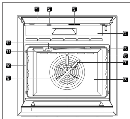
obr. 4.1 Uspořádání – část 1
