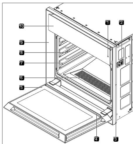
obr. 4.2 Uspořádání – část 2
