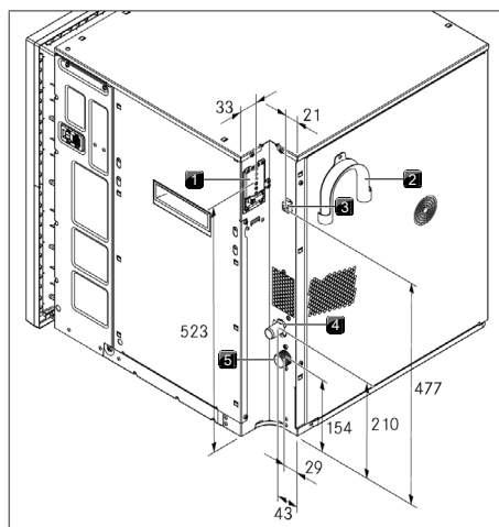
obr. 8.10 Přípojky zařízení
