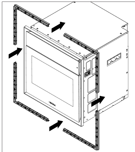
obr. 8.6 Demontáž distančního rámu
