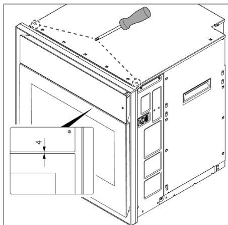
obr. 8.15 Nastavení vzdálenosti ovládací jednotky a dvířek
