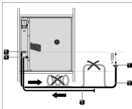
obr. 8.11 Odvod vody
