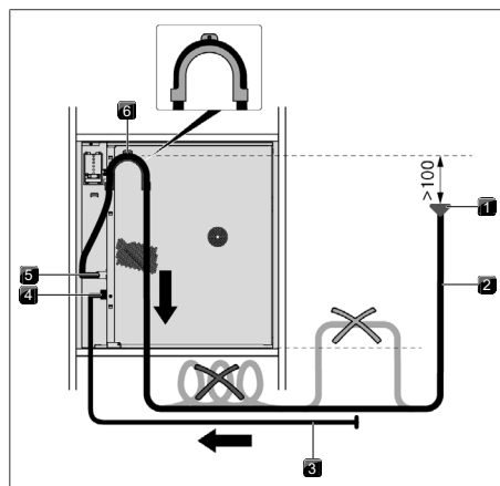
obr. 8.12 Odvod vody přes přidržené kolínko
