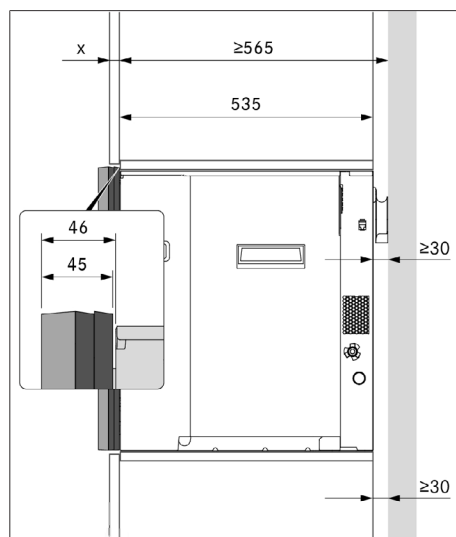
obr. 8.5 Montážní rozměry se 2 distančními rámy
