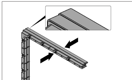
obr. 8.7 2 prvky distančního rámu
