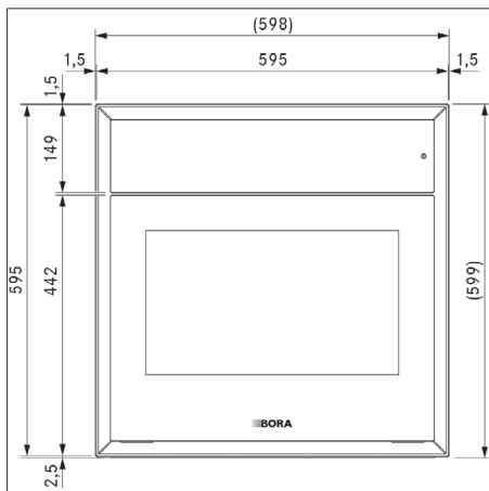
obr. 3.1 Pohled zepředu na spotřebič XBO
