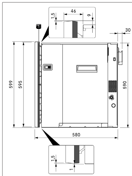
obr. 8.2 Rozměry
