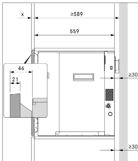
obr. 8.3 Montážní rozměry bez distančního rámu
