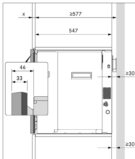
obr. 8.4 Montážní rozměry s 1 distančním rámem
