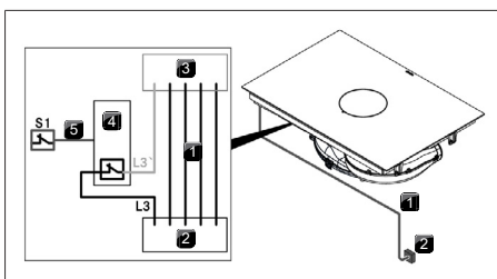
Fig. 10.26 Tilslutningsdiagram med ekstern omkoblingskontakt
