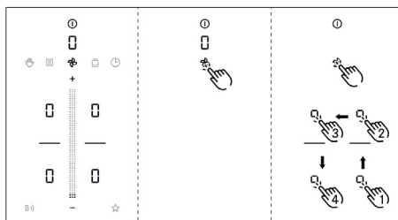
Fig. 10.31 Visning af Forhandler- og servicemenu i displayet
