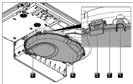
Fig. 8.3 Luftføringskabinettet
