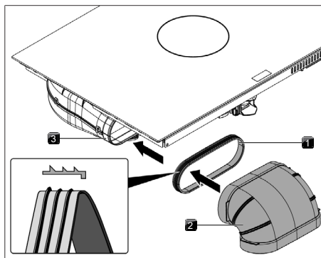
Fig. 10.24 Tilslutning til kanalsystem
