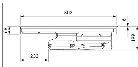
Fig. 3.5 PUXU2/R - enhedens mål set forfra
