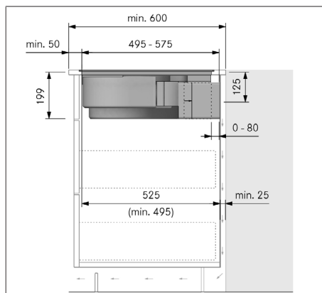
Fig. 10.13 Indbygningsmål ved recirkulationsluft, monteringsvariant A
