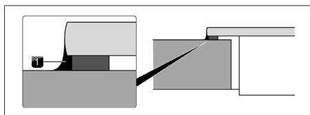
Fig. 10.35 Silikonemasse ved overflademontering
