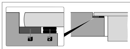
Fig. 10.22 Højdeudligningsplader
