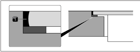
Fig. 10.36 Silikonetætningsmasse ved planimet montering
