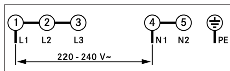
Fig. 10.28 Tilslutningsskema, 1-faset tilslutning
