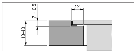
Fig. 10.6 Falsmål til planlimet montering
