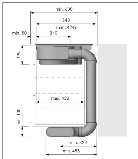
Fig. 10.9 Indbygningsmål aftræk, dybde i køkkenbord 600 mm
