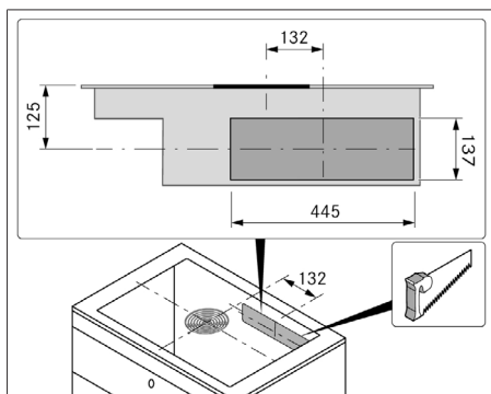
Fig. 10.11 Udskæring i bagvæggen
