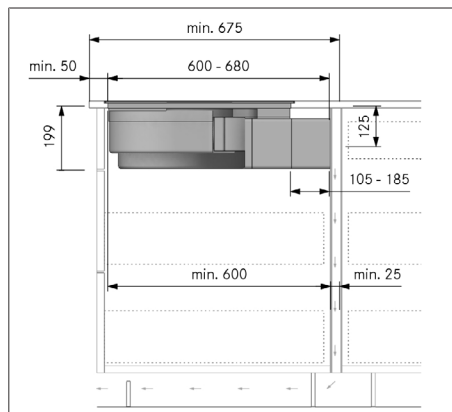
Fig. 10.14 Indbygningsmål ved recirkulationsluft-monteringsvariant A, dybde i køkkenbord 675 mm
