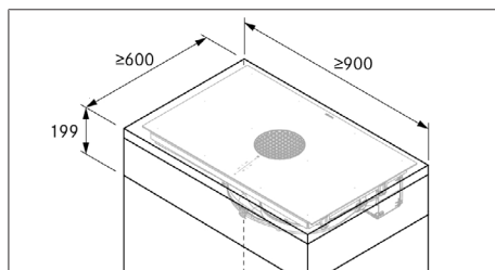
Fig. 10.4 Møbel mindstemål X Pure
