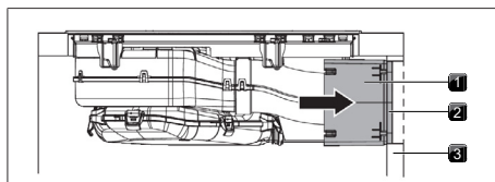
Fig. 10.25 Tilslutning til bagvæggen
