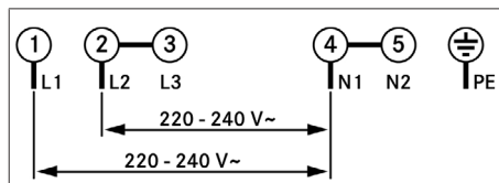
Fig. 10.29 Tilslutningsskema, 2-faset tilslutning
