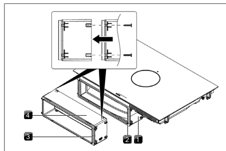
Fig. 10.15 Forlængelse af teleskopudtrækket
