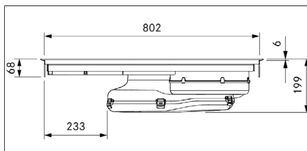
Fig. 3.2 PUXA2/R - enhedens mål set forfra
