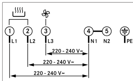
Fig. 10.27 Tilslutningsskema, 3-faset tilslutning
