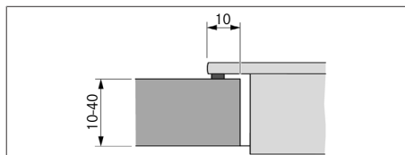
Fig. 10.8 Monteringsmål til overflademontering
