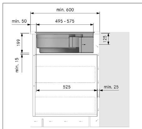
Fig. 10.16 Indbygningsmål ved recirkulationsluft-monteringsvariant B, dybde i køkkenbord 600 mm
