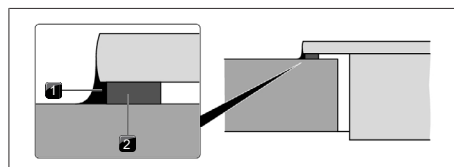
Fig. 10.17 Forseglingsstape ved overflademontering
