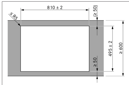
Fig. 10.7 Udskæringsmål til overflademontering
