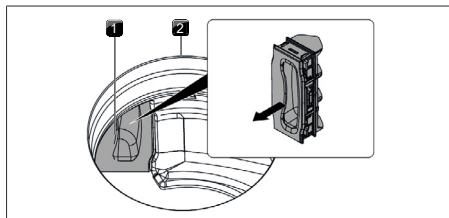
Fig. 8.4 Udtagning af filterudskiftningsklap
