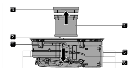
Fig. 10.20 Indsætning af kogepladen i midten
