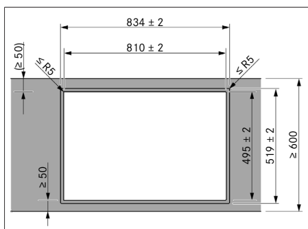
Fig. 10.5 Udskæringsmål til planlimet montering
