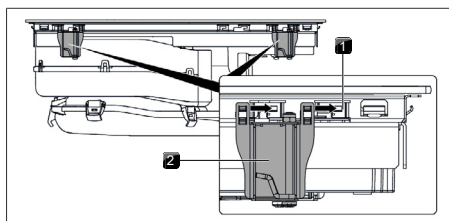
Fig. 10.19 Anbringelse af monteringsklemmer
