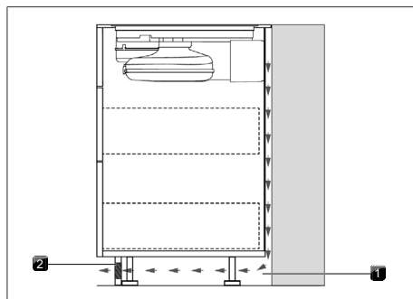
Fig. 10.10 Returstrømsåbning i sokkelområdet
