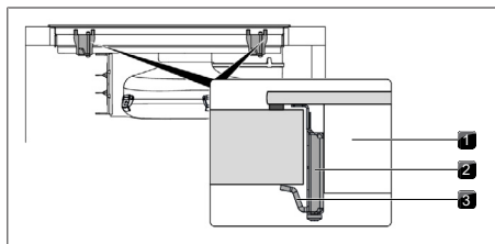
Fig. 10.23 Fastgøring af kogepladen i midten
