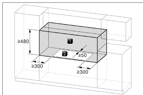
Fig. 10.3 Krævet frirum
