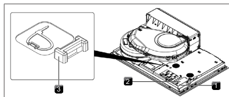
Fig. 10.30 Elektriske tilslutninger til kogepladen
