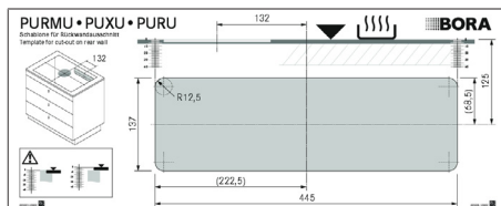
Fig. 10.12 Skabelon til udskæring i bagvæggen
