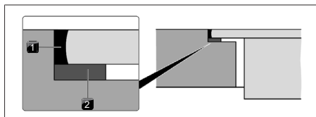
Fig. 10.18 Forseglingsstape til planlimet montering
