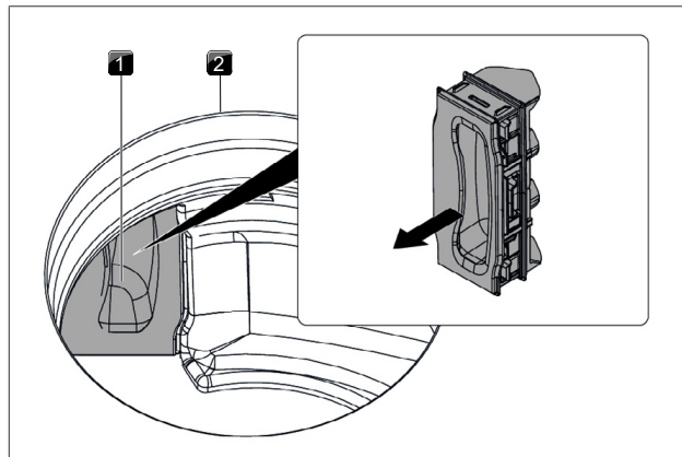
obr. 7.6 Sejmutí výměnné klapky filtru
