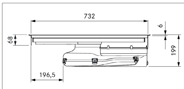
obr. 3.11 Rozměry spotřebiče PURU – pohled zepředu
