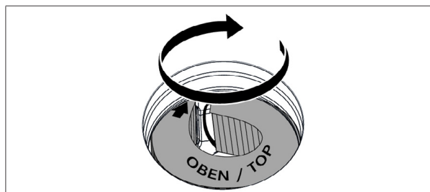
obr. 7.11 Úprava filtru s aktivním uhlím do správné polohy
