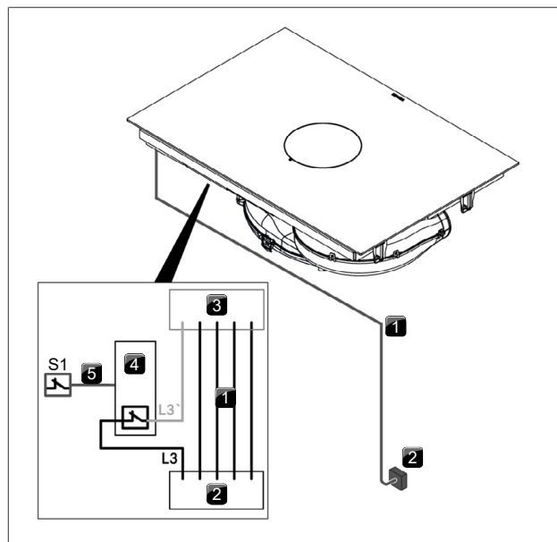
obr. 9.38 Schéma zapojení s externím spínacím kontaktem
