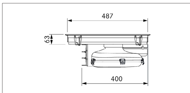
obr. 3.9 Rozměry spotřebiče PURA – pohled z boku
