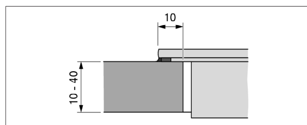
obr. 9.9 Rozměry podkladu pro montáž na povrch
