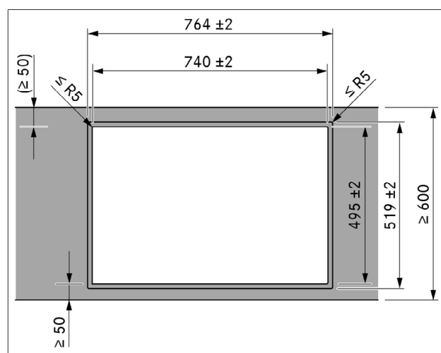
obr. 9.10 Rozměry výřezu pro plošně zarovnanou montáž
