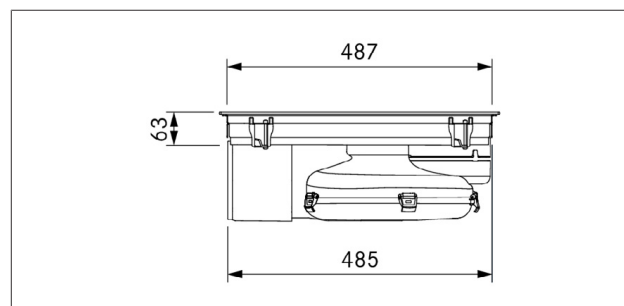
obr. 3.12 Rozměry spotřebiče PURU – pohled z boku
