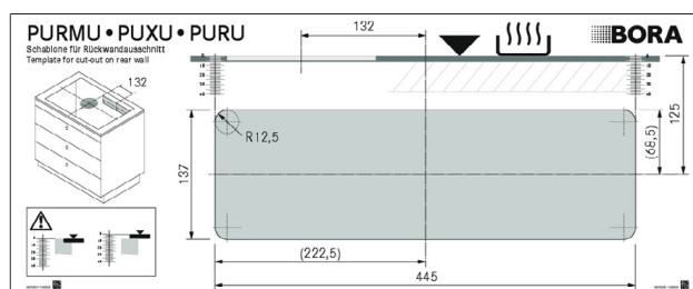
obr. 9.25 Šablona pro výřez zadní stěny
