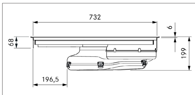
obr. 3.8 Rozměry spotřebiče PURA – pohled zepředu
