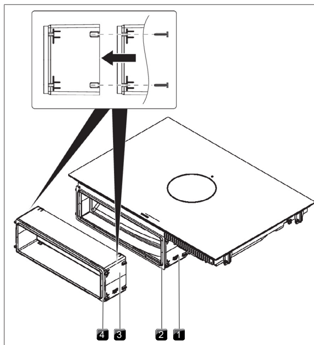
obr. 9.32 Nadstavení teleskopického výsuvu
