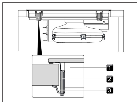
obr. 9.36 Upevnění varné desky do středu
