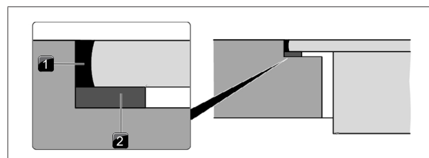
obr. 9.29 Těsnicí páska při plošně zarovnané montáži
