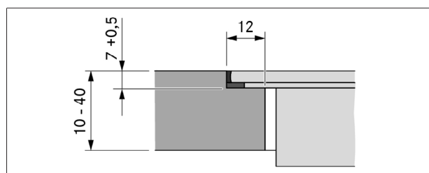
obr. 9.7 Rozměr drážky pro plošně zarovnanou montáž
