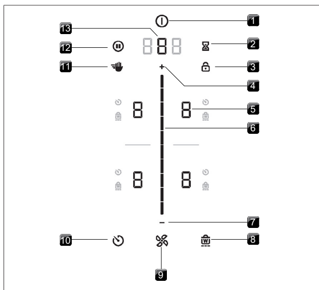
obr. 4.5 Dotykové oblasti / tlačítka
