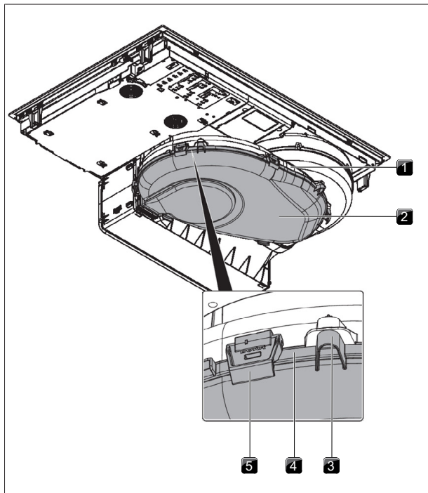
obr. 7.5 Skříň ventilace
