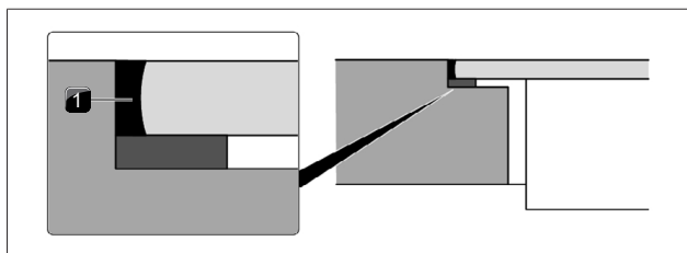
obr. 9.48 Silikonová těsnicí hmota při plošně zarovnané montáži
