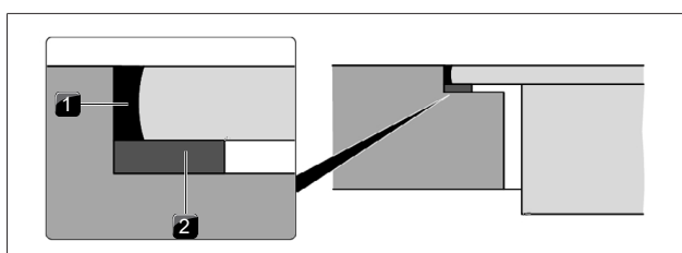
obr. 9.16 Těsnicí páska při plošně zarovnané montáži
