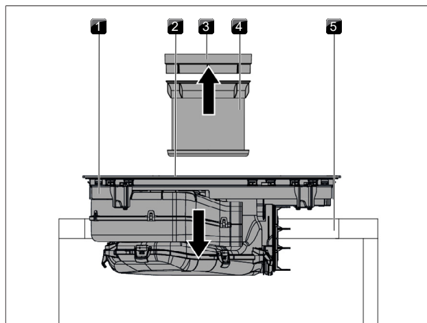
obr. 9.18 Upevnění varné desky do středu
