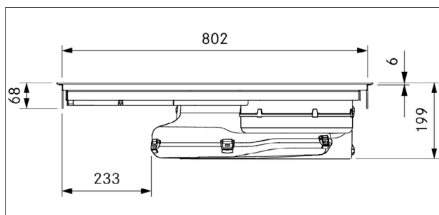
obr. 3.5 Rozměry spotřebiče PUXU – pohled zepředu
