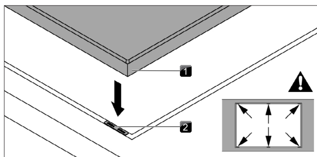
obr. 9.19 Pozice podložek k nastavení výšky
