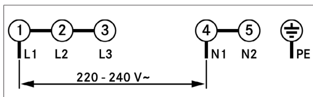
obr. 9.40 Schéma zapojení 1fázové přípojky
