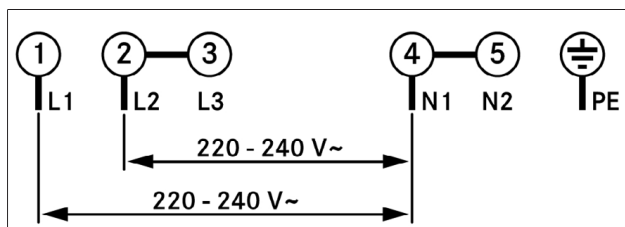
obr. 9.41 Schéma zapojení 2fázové přípojky
