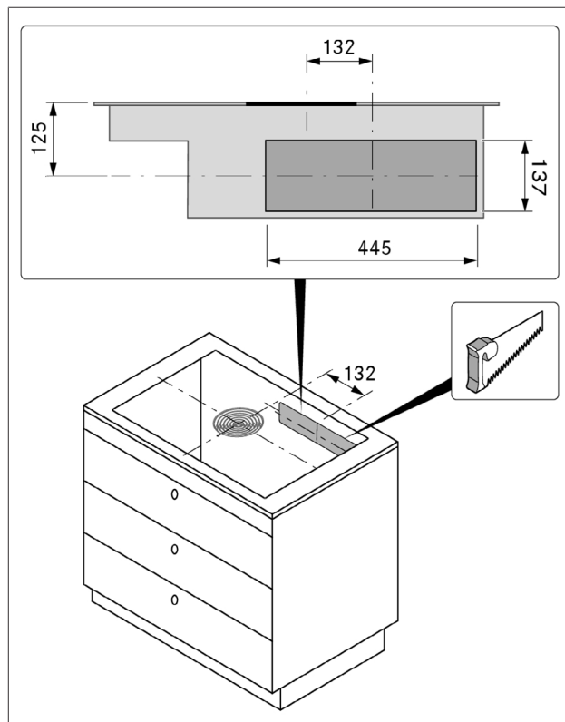
obr. 9.24 Výřez v zadní stěně
