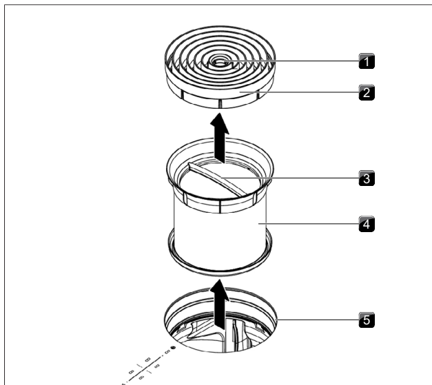
obr. 7.3 Demontáž součástí
