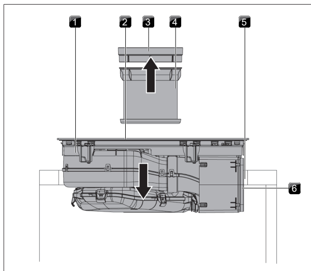
obr. 9.33 Upevnění varné desky do středu
