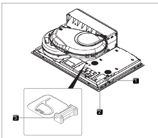
obr. 9.42 Elektrické přípojky varné desky
