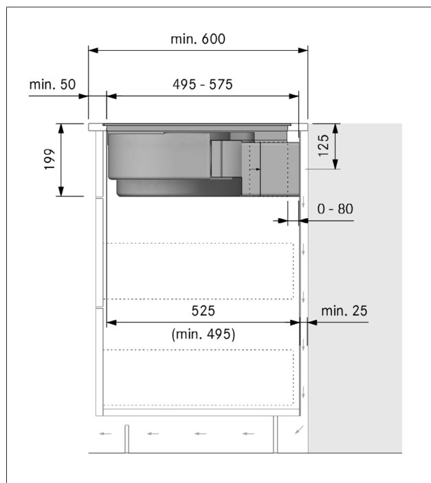
obr. 9.26 Rozměry montáže u recirkulujícího vzduchu, varianta montáže A
