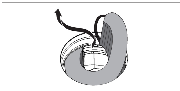
obr. 7.8 Vyjmutí filtru s aktivním uhlím z otvoru přívodní trysky
