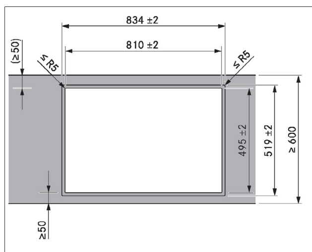
obr. 9.6 Rozměry výřezu pro plošně zarovnanou montáž
