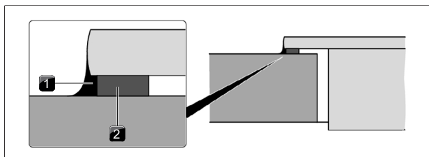
obr. 9.15 Těsnicí páska při montáži na povrch
