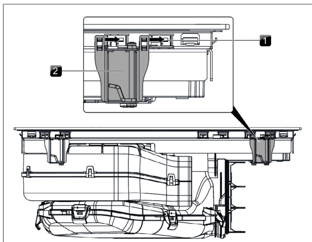
obr. 9.17 Umístění montážních svorek
