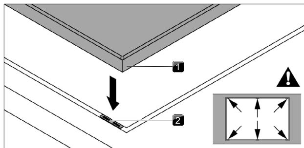
obr. 9.34 Pozice podložek k nastavení výšky
