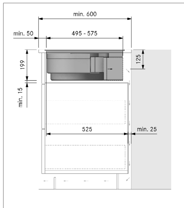
obr. 9.27 Rozměry montáže u varianty montáže B, hloubka pracovní desky 600 mm
