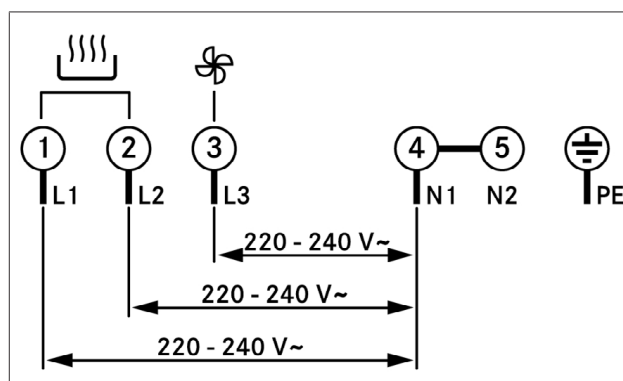
obr. 9.39 Schéma zapojení 3fázové přípojky
