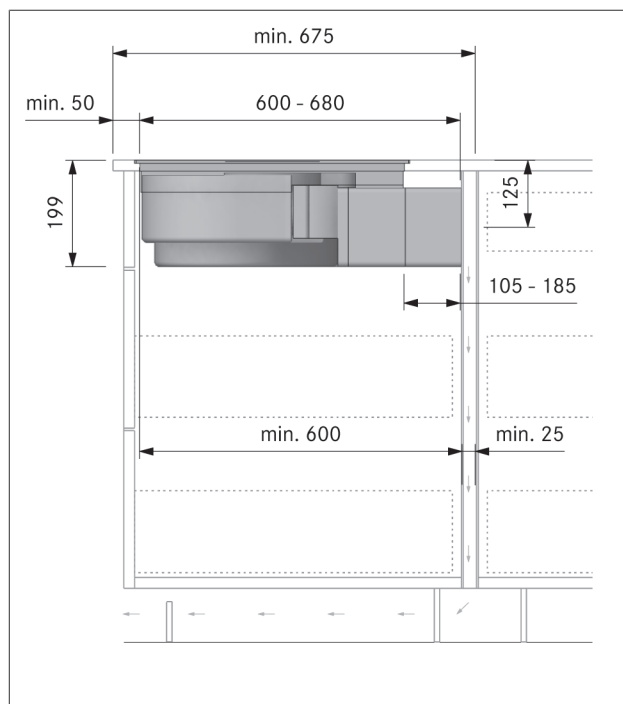
obr. 9.31 Rozměry montáže u varianty montáže A, hloubka pracovní desky od 675 mm
