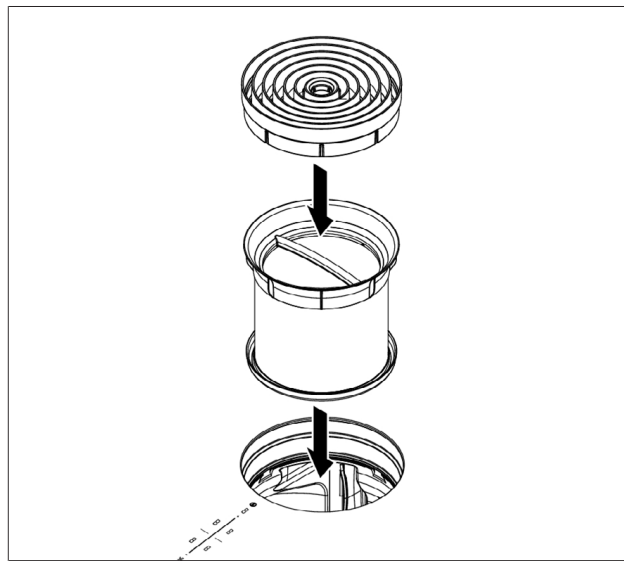
obr. 7.4 Montáž součástí
