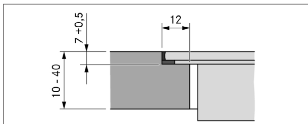
obr. 9.11 Rozměr drážky pro plošně zarovnanou montáž
