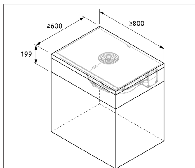
obr. 9.5 Minimální rozměry nábytku – Pure
