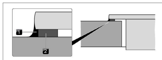
obr. 9.28 Těsnicí páska při montáži na povrch
