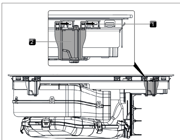
obr. 9.30 Umístění montážních svorek
