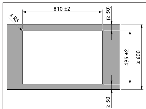
obr. 9.8 Rozměry výřezu pro montáž na povrch
