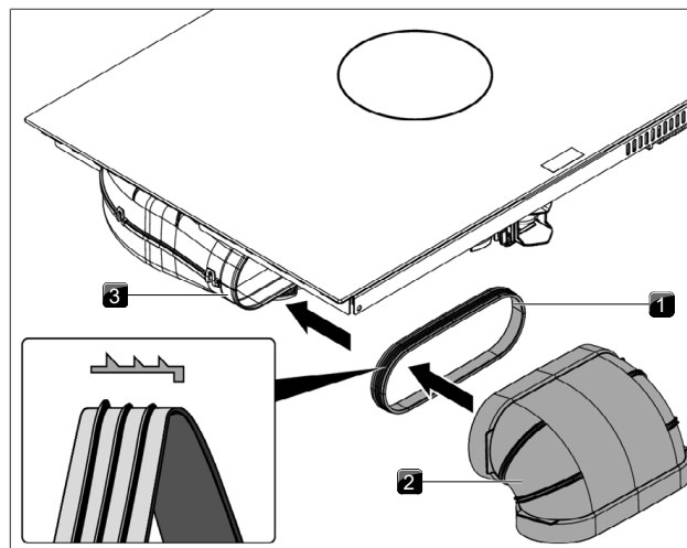
obr. 9.22 Připojení systému odtahových potrubí
