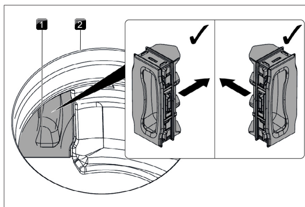
obr. 7.12 Nasazení výměnné klapky filtru
