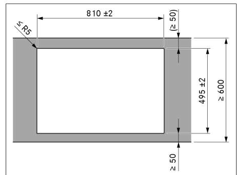
Bild 9.8 Utskärningsmått för ytmonteringen
