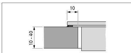
Bild 9.13 Pålsettningsmått för ytmonteringen
