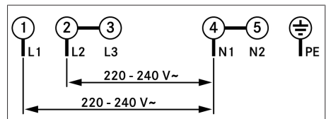
Bild 9.41 Anslutningsschema 2-fas anslutning
