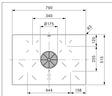
Bild 3.7 PURA apparatmått bild från ovan
