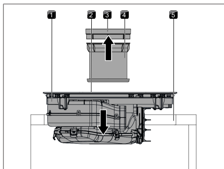
Bild 9.18 Placera spishällen centrerat
