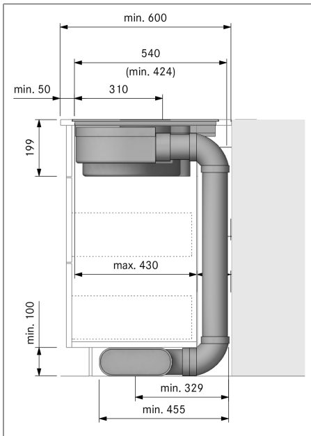
Bild 9.14 Inbyggnadsmått frånluft, bänkskivans djup 600 mm
