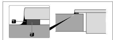
Bild 9.28 Tätningsband vid ytmontering
