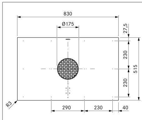
Bild 3.4 PUXU apparatmått bild från ovan
