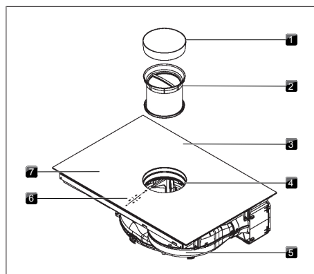
Bild 4.1 Uppbyggnad
