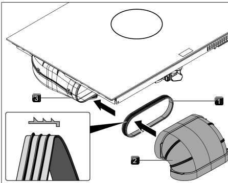
Bild 9.22 Anslutning till kanalsystemet
