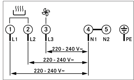
Bild 9.39 Anslutningsschema 3-fas anslutning
