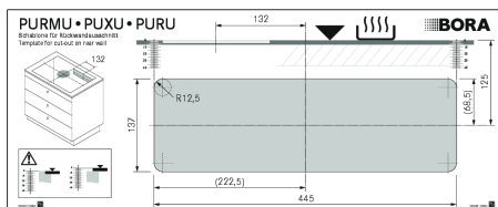
Bild 9.25 Schablone für öppningen i den bakre väggen
