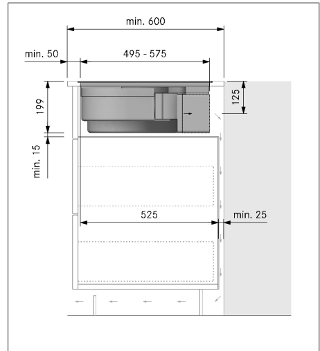
Bild 9.27 Inbyggadsmått vid luftcirkulation monteringsvariant B, bänkskivans djup 600 mm
