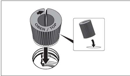
Bild 7.10 Sätta in aktivkolfiltret i utsugningsöppningen
