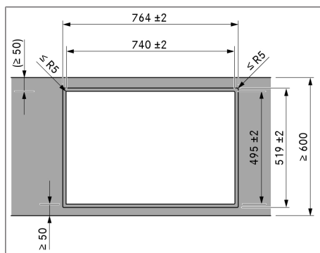
Bild 9.10 Utskärningsmått för planmontering
