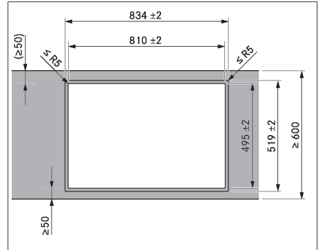
Bild 9.6 Utskärningsmått för planmontering
