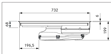
Bild 3.8 PURA apparatmått bild framifrån
