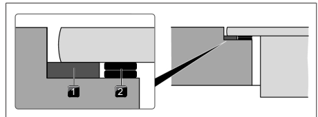
Bild 9.35 Höjdutjämningsplattor
