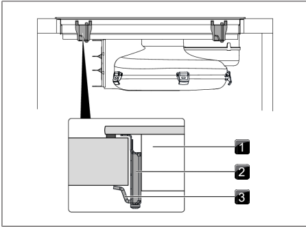
Bild 9.21 Fästa spishällen centrerat
