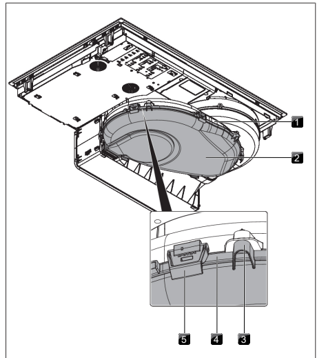
Bild 7.5 Luftledningskåpa
