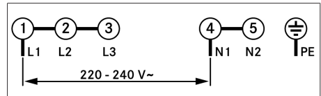
Bild 9.40 Anslutningsschema 1-fas anslutning
