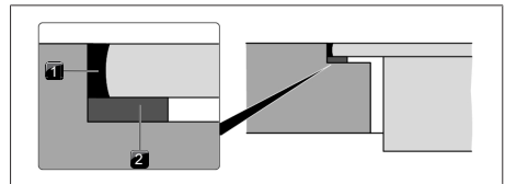
Bild 9.16 Tätningsband vid planmontering
