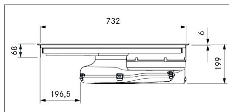
Bild 3.11 PURU apparatmått bild framifrån
