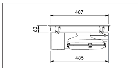
Bild 3.12 PURU apparatmått bild från sidan
