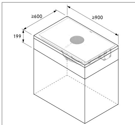
Bild 9.4 Möbelns minimimått X Pure
