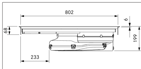
Bild 3.5 PUXU apparatmått bild framifrån
