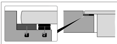
Bild 9.20 Höjdutjämningsplattor
