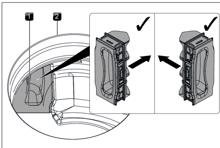
Bild 7.12 Sätta i filterbytesklaffen
