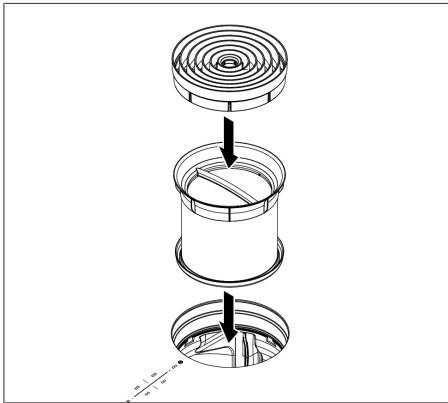
Bild 7.4 Montering av komponenterna
