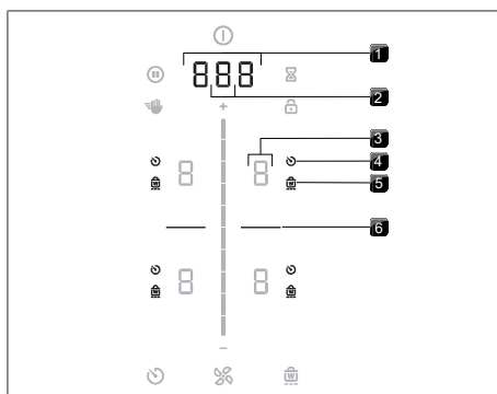
Bild 4.6 Display-områden
