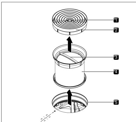
Bild 7.3 Avmontering av komponenterna
