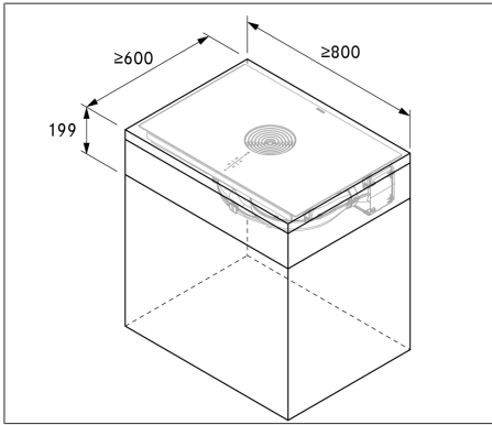
Bild 9.5 Möbelns minimimått Pure
