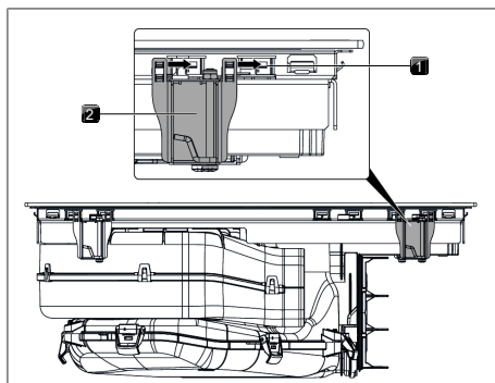
Bild 9.30 Sätta på monteringsklämmorna
