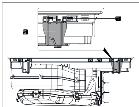
Bild 9.17 Sätta på monteringsklämmorna
