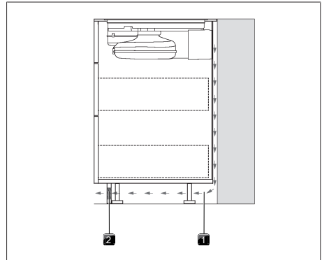
Bild 9.23 Återströmningsöppning i sockelområdet
