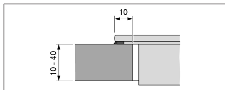
Bild 9.9 Pålsettningsmått för ytmonteringen
