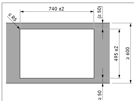
Bild 9.12 Utskärningsmått för ytmonteringen
