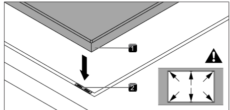
Bild 9.34 Höjdutjämningsplattornas positionering
