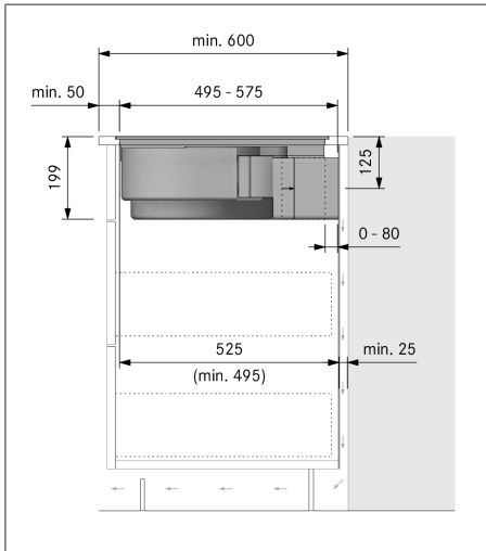
Bild 9.26 Inbyggadsmått vid luftcirkulation, monteringsvariant A
