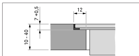
Bild 9.11 Fälsmått för planmontering
