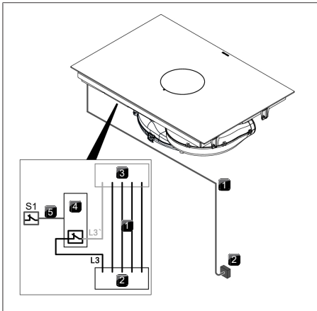
Bild 9.38 Anslutningsschema med extern kontakt
