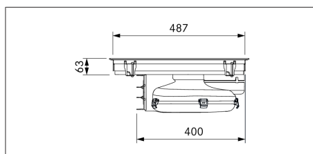
Bild 3.9 PURA apparatmått bild från sidan
