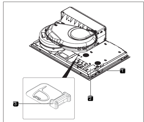
Bild 9.42 Spishällens elektriska anslutningar
