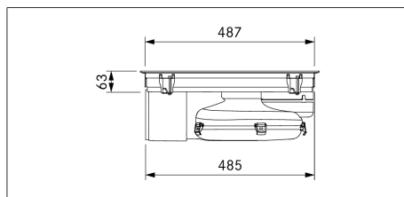
Bild 3.6 PUXU apparatmått bild från sidan
