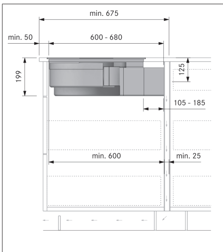
Bild 9.31 Inbyggningmått vid luftcirkulation monteringsvariant A, bänkskivans djup från 675 mm
