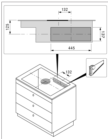
Bild 9.24 Utskärning i den bakre väggen
