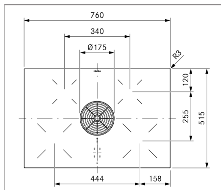
Bild 3.10 PURU apparatmått bild från ovan
