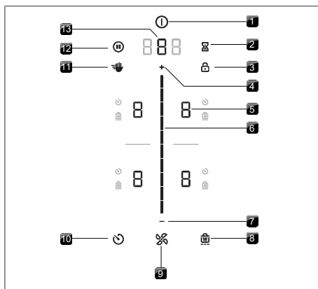
Bild 4.5 Touch-områden/knappar
