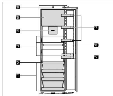
Rys. 5.2 Budowa C178KGF
