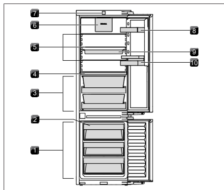
Rys. 5.4 Budowa C178KGW
