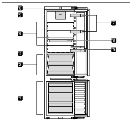
Rys. 5.5 Budowa C194KG
