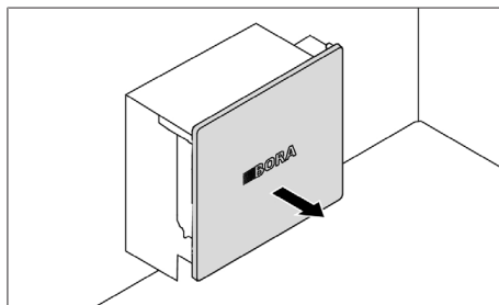
Rys. 10.1 Wyjmowanie pokrywy wentylatora z mocowaniem filtra zapachów
