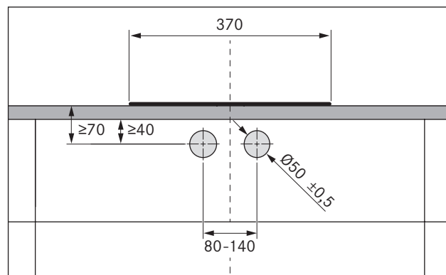
Fig. 5.8 Drill template
