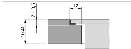
Fig. 10.6 Medida del rebaje para un montaje enrasado
