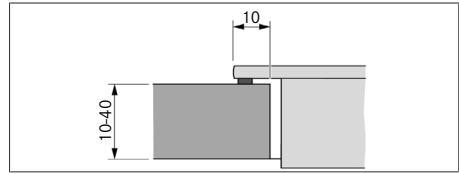
Fig. 10.8 Medida del apoyo para montaje superpuesto
