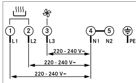
Fig. 10.27 Esquema de conexiones, conexión trifásica
