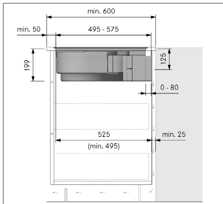
Fig. 10.13 Medidas de montaje con recirculación, variante de montaje A
