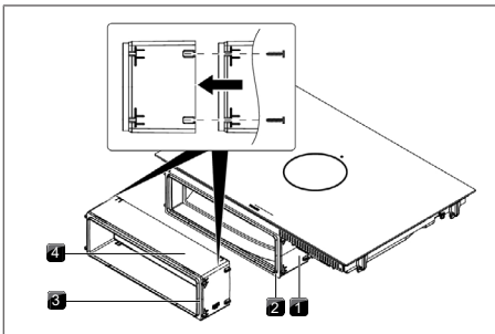
Fig. 10.15 Prolongación de la extensión telescópica
