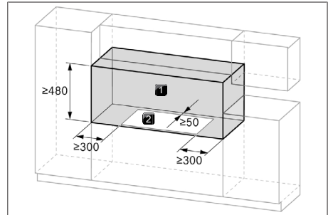
Fig. 10.3 Espacio libre requerido
