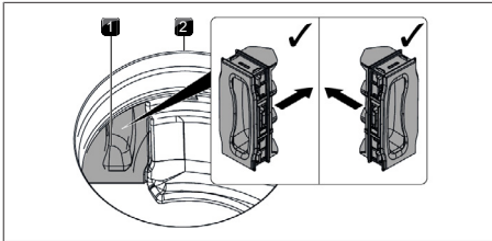
Fig. 8.10 Colocación de la trampilla para el cambio del filtro
