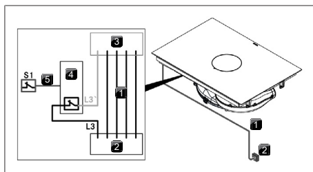
Fig. 10.26 Esquema de conexiones con contacto de conmutación externo
