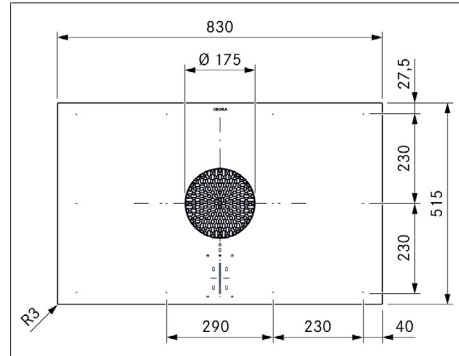
Fig. 3.1 PUXA2/R dimensiones, vista superior
