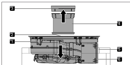
Fig. 10.20 Colocación de la placa de cocción en posición centrada
