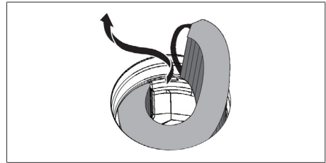
Fig. 8.6 Extracción del filtro de carbón activo de la abertura de entrada
