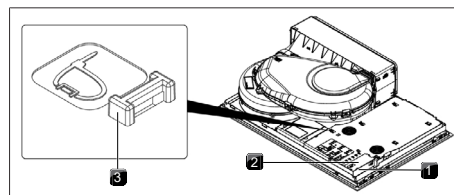
Fig. 10.30 Conexiones eléctricas de la placa de cocción
