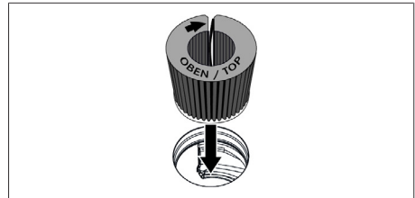
Fig. 8.8 Colocación del filtro de carbón activo en la abertura del extractor
