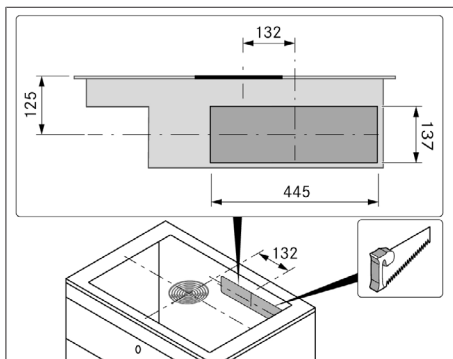
Fig. 10.11 Recorte del panel trasero
