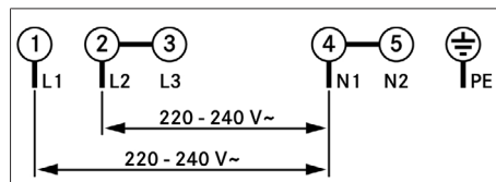
Fig. 10.29 Esquema de conexiones, conexión bifásica
