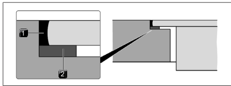
Fig. 10.18 Cinta selladora para montaje enrasado
