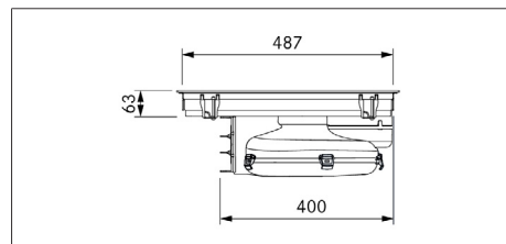
Fig. 3.3 PUXA2/R dimensiones, vista lateral
