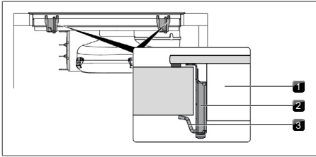
Fig. 10.23 Fijación de la placa de cocción en posición centrada
