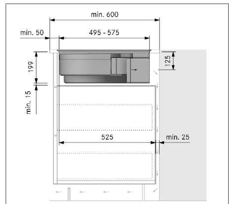
Fig. 10.16 Medidas de montaje para la variante de recirculación B, profundidad de la encimera 600 mm
