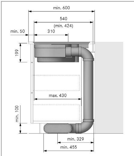
Fig. 10.9 Medidas de montaje extracción al exterior, profundidad de la encimera 600 mm
