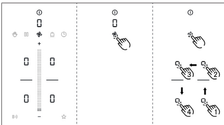
Fig. 10.31 Acceso a la pantalla del menú de distribuidores y de servicio
