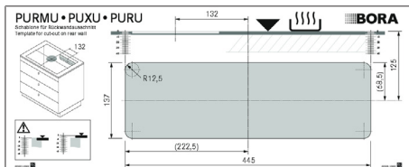
Fig. 10.12 Plantilla para el recorte del panel trasero
