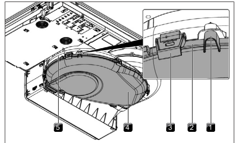
Fig. 8.3 Carcasa de conducción del aire
