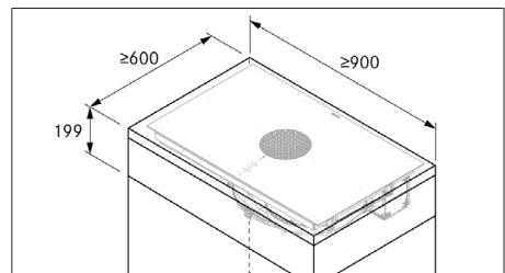
Fig. 10.4 Medidas mínimas de los muebles X Pure
