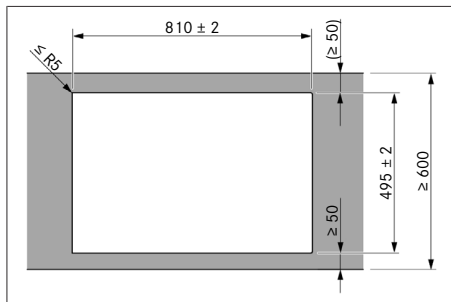
Fig. 10.7 Medidas del recorte para montaje superpuesto
