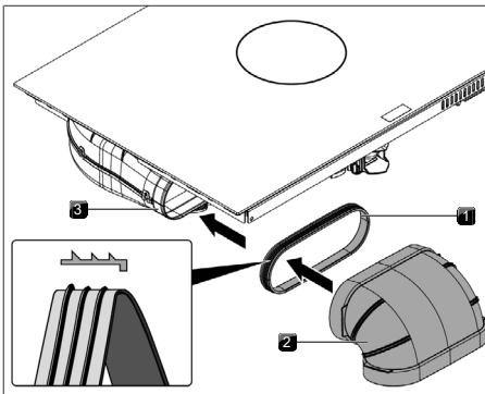
Fig. 10.24 Conexión al sistema de conductos
