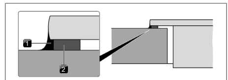
Fig. 10.17 Cinta selladora para montaje superpuesto
