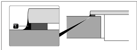
Fig. 10.35 Silicona de sellado para montaje superpuesto
