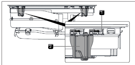
Fig. 10.19 Colocación de las abrazaderas de montaje
