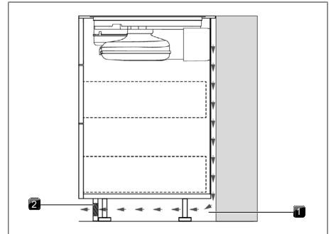
Fig. 10.10 Abertura de flujo de retorno en la zona del zócalo
