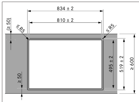
Fig. 10.5 Medidas del recorte para montaje enrasado
