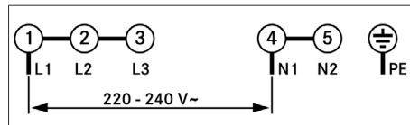
Fig. 10.28 Esquema de conexiones, conexión monofásica
