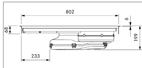
Fig. 3.2 PUXA2/R dimensiones, vista frontal
