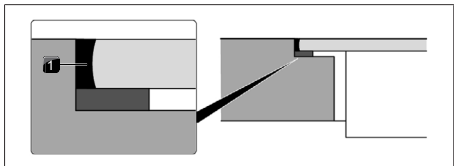
Fig. 10.36 Silicona de sellado para montaje enrasado
