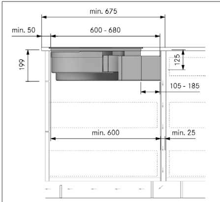
Fig. 10.14 Medidas de montaje para la variante de recirculación A, profundidad de la encimera 675 mm o más
