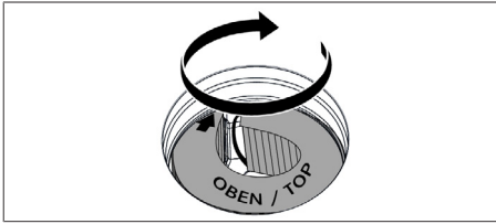
Fig. 8.9 Colocación del filtro de carbón activo en la posición final
