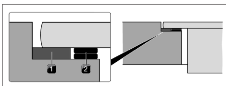
Fig. 10.22 Placas de compensación de altura
