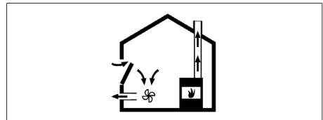
Fig. 10.2 Instalación de la extracción al exterior – correcta
