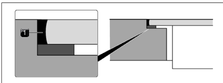
Abb. 10.36 Silikondichtmasse bei flächenbündiger Montage
