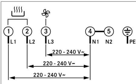
Abb. 10.27 Anschlusschema 3-Phasen-Anschluss
