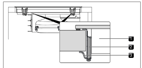
Abb. 10.23 Kochfeld mittig befestigen
