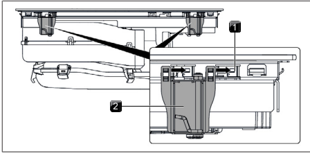
Abb. 10.19 Montageklappen anbringen
