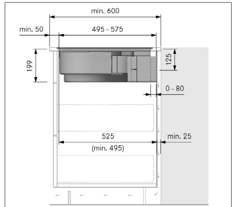
Abb. 10.13 Einbaumaße bei Umluft, Montagevariante A
