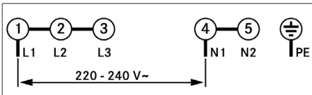
Abb. 10.28 Anschlusschema 1-Phasen-Anschluss
