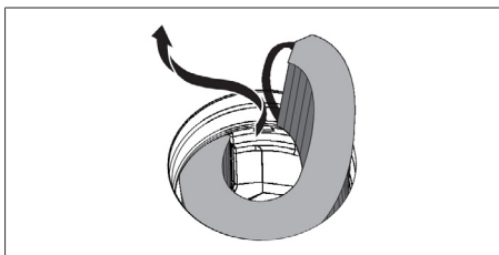
Abb. 8.6 Aktivkohlefilter aus der Einströmöffnung entnehmen
