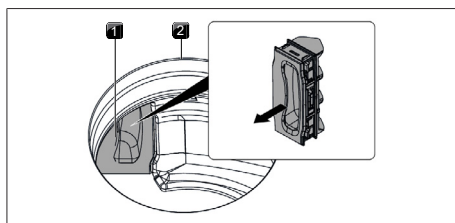
Abb. 8.4 Filterwechsellappe entfernen
