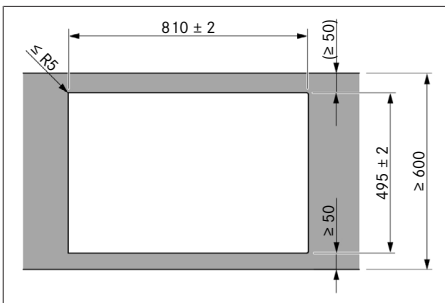
Abb. 10.7 Ausschnittsmaße für Aufsatzmontage
