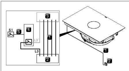
Abb. 10.26 Anschlusschema mit externem Schaltkontakt
