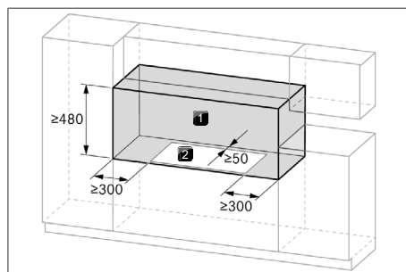
Abb. 10.3 Erforderlicher Freiraum
