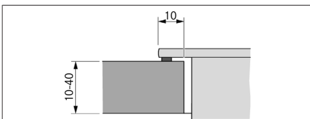
Abb. 10.8 Auflagemaß für Aufsatzmontage
