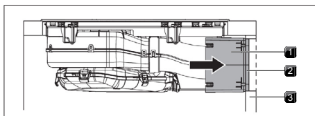
Abb. 10.25 Rückwandanschluss
