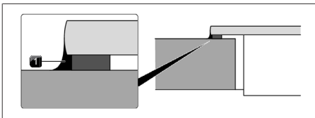
Abb. 10.35 Silikondichtmasse bei Aufsatzmontage
