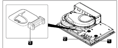
Abb. 10.30 Elektrische Anschlüsse des Kochfeldes
