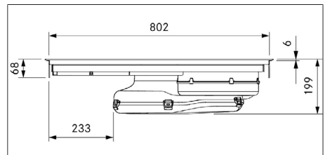
Abb. 3.2 PUXA2/R Gerätemaße Vorderansicht
