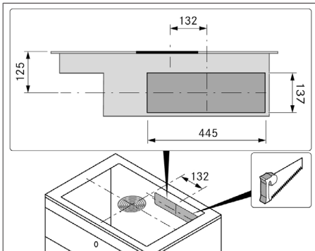
Abb. 10.11 Rückwand-Ausschnitt
