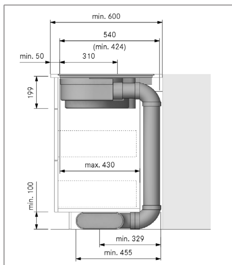
Abb. 10.9 Einbaumaße Abluft, Arbeitsplattentiefe 600 mm
