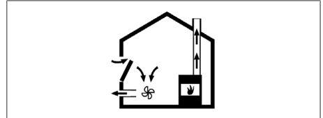
Abb. 10.2 Abluftmontage – korrekt
