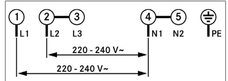
Abb. 10.29 Anschlusschema 2-Phasen-Anschluss
