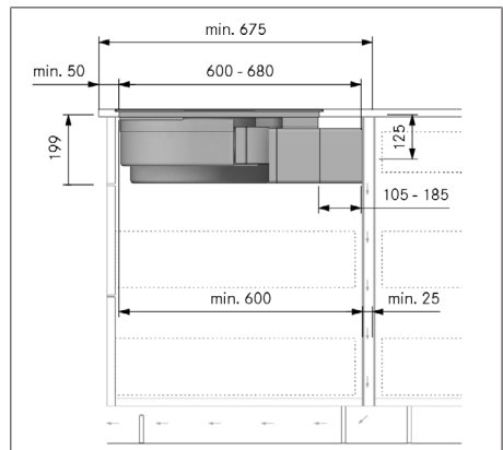
Abb. 10.14 Einbaumaße bei Umluft-Montagevariante A, Arbeitsplattentiefe ab 675 mm
