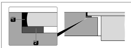
Abb. 10.18 Dichtungsband bei flächenbündiger Montage
