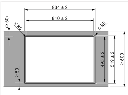
Abb. 10.5 Ausschnittsmaße für flächenbündige Montage
