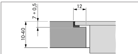
Abb. 10.6 Falzmaß für flächenbündige Montage
