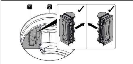
Abb. 8.10 Filterwechselklappe einsetzen
