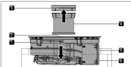
Abb. 10.20 Kochfeld mittig einsetzen
