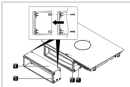
Abb. 10.15 Verlängerung des Teleskopauszuges
