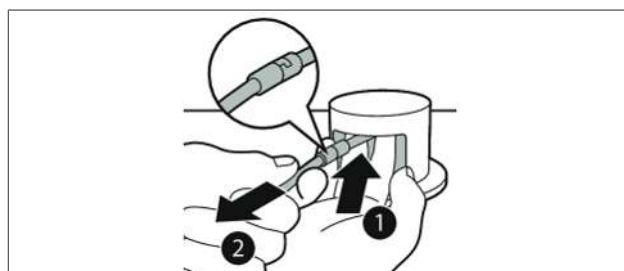
Kuva 6.2 Tyhjiöintiletkun liitoksen irrottaminen
