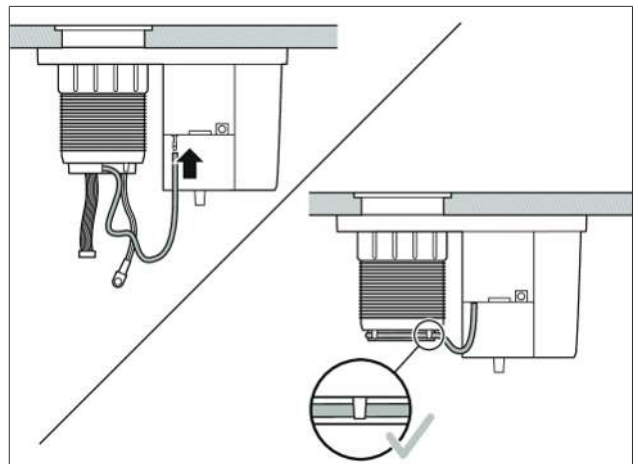
Kuva 8.17 Tyhjiöintiletkun liittäminen ja kiinnittäminen kiinnikkeillä
