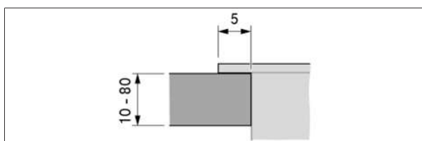
Fig. 8.5 Dimensjoner overflatemontering
