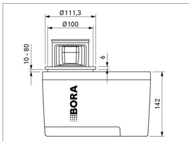
Fig. 3.1 Visning forfra QVac
