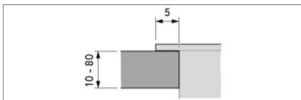
Rys. 8.5 Wymiar montażu elementu z uskokiem
