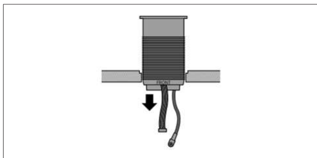
Rys. 8.13 Wkładanie modułu pop-up
