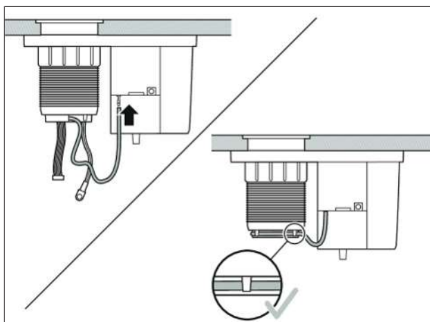
Obr. 8.17 Prípojenie vákuovacej hadice a jej upevnenie držiakmi
