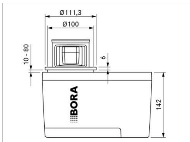
Obr. 3.1 Pohľad spredu na QVac
