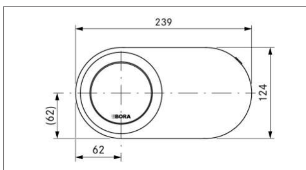
Obr. 3.2 Pohľad zhora na QVac
