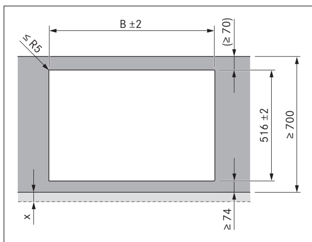
Obr. 5.5 Rozmery výrezu pre montáž na povrch
