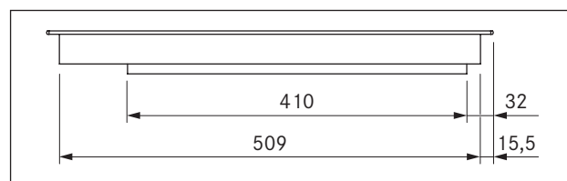
Obr. 3.4 Rozmery varnej dosky PKI11, pohľad z boku
