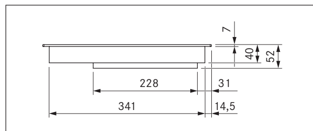
Obr. 3.3 Rozmery varnej dosky PKI11, pohľad spredu
