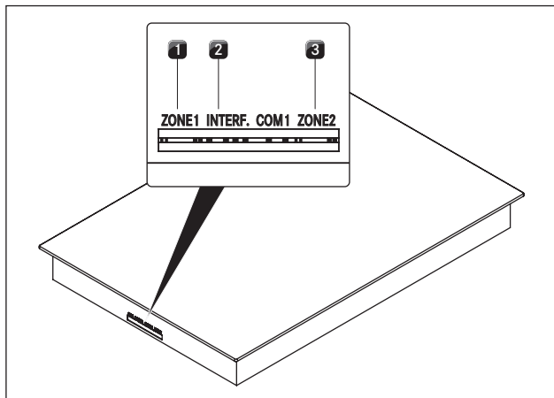
Obr. 5.18 Pripojky na varnej doske
