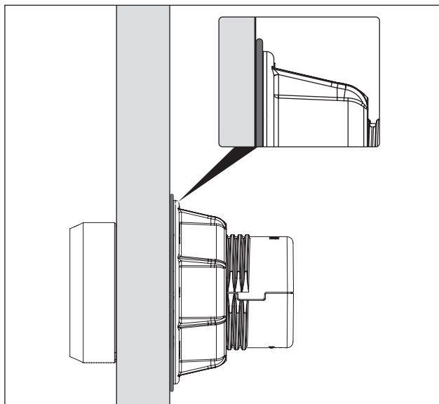
Fig. 5.14 Ferdig montert bølgefjær
