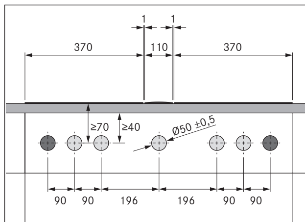
Fig. 5.15 Frontplateborehull for 2 platetopper og 1 avtrekk
