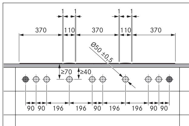
Fig. 5.16 Frontplateborehull for 3 platetopper og 2 avtrekk
