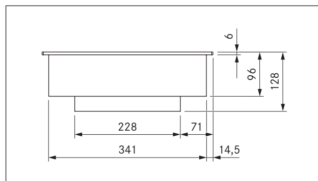
Fig. 3.3 PKIW1 apparatmål visning forfra
