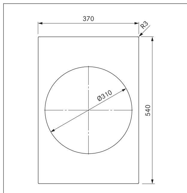
Fig. 3.2 PKIW1 apparatmål visning ovenfra
