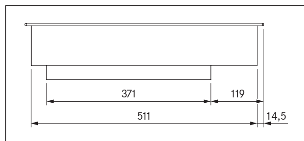
Fig. 3.4 PKIW1 apparatmål visning fra siden
