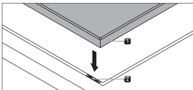
Fig. 5.18 Platetopp og høydejusteringsplater
