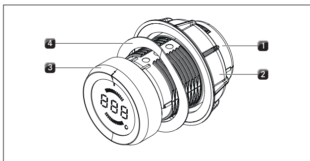
Fig. 5.12 Oppbygning betjeningsknott
