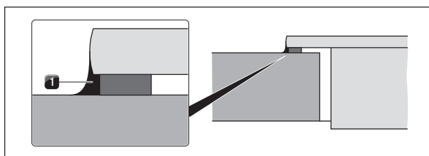
Fig. 5.24 Silikonfugemasse ved overflatemontering
