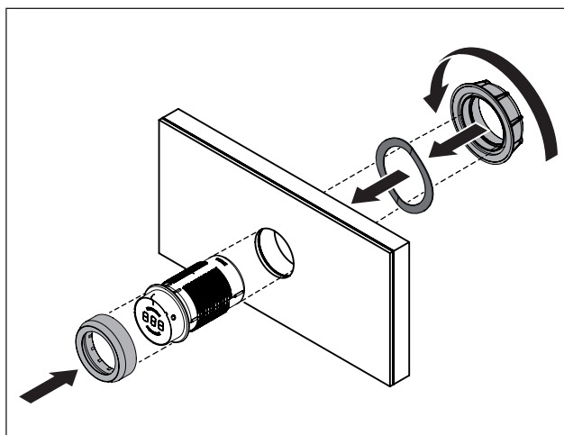
Fig. 5.13 Montere betjeningsknott
