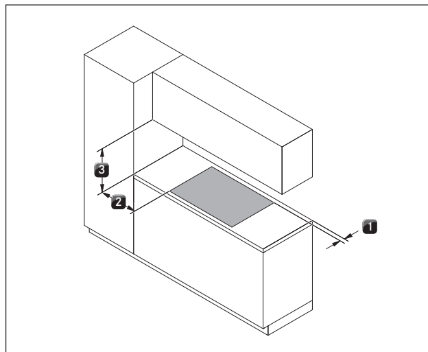
Fig. 5.1 Minimumsavstander
