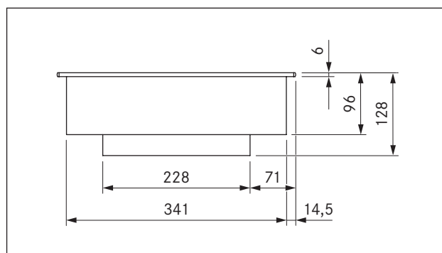
Obr. 3.3 Rozmery varnej dosky PKIW1, pohľad spredu
