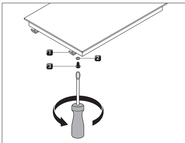
Obr. 5.19 Upevňovacie svorky
