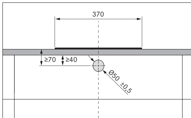
Obr. 5.11 Vŕtacia šablóna
