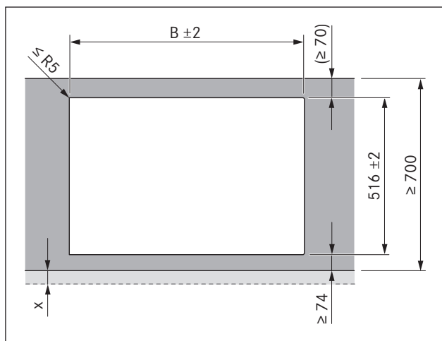
Obr. 5.5 Rozmery výrezu pre montáž na povrch
