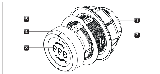
Obr. 4.2 Konštrukcia ovládacieho kolieska
