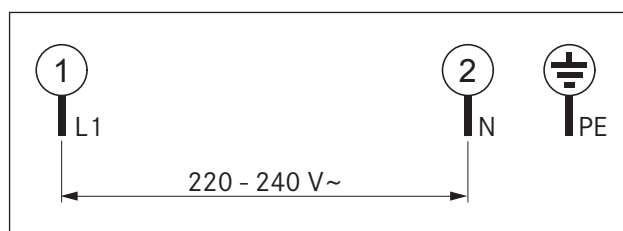
Obr. 5.23 Schéma zapojenia 1-fázové
