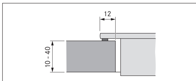
Obr. 5.6 Rez montážou na povrch
