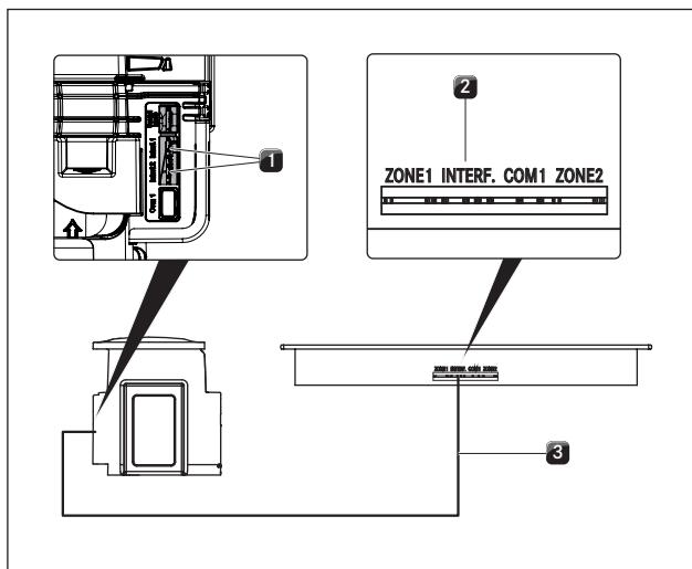
Obr. 5.22 Prípojka odťahovej automatiky
