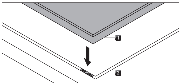
Obr. 5.18 Varná doska a podložky na nastavenie výšky
