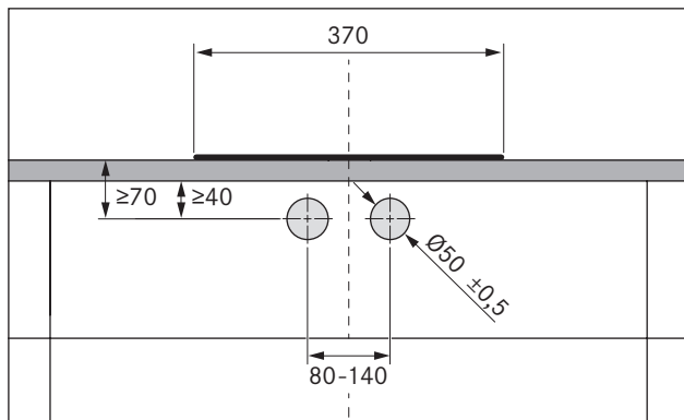
Obr. 5.9 Vŕtacia šablóna
